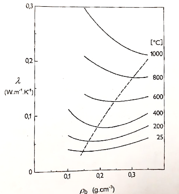
Obr. 9 Závislost tepelné vodivosti rohoží a desek. [4]
