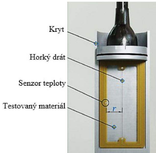
Obr. 3 Schéma metody topného drátu. [7]
