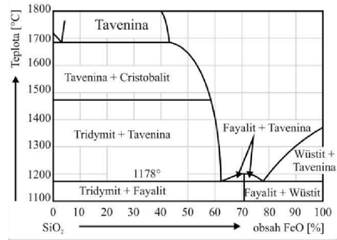
Obr. 17 Rovnovážný diagram SiO 2 -FeO. [33]
