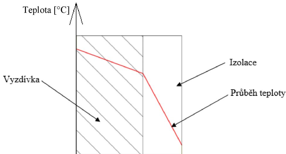
Obr. 15 Schéma průběhu teploty přes stěnu pece.
