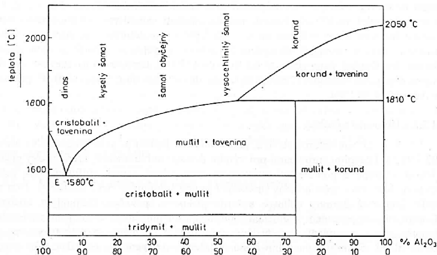
Obr. 6 Rovnovážný diagram \text{SiO}_2\text{-Al}_2\text{O}_3 . [12]
