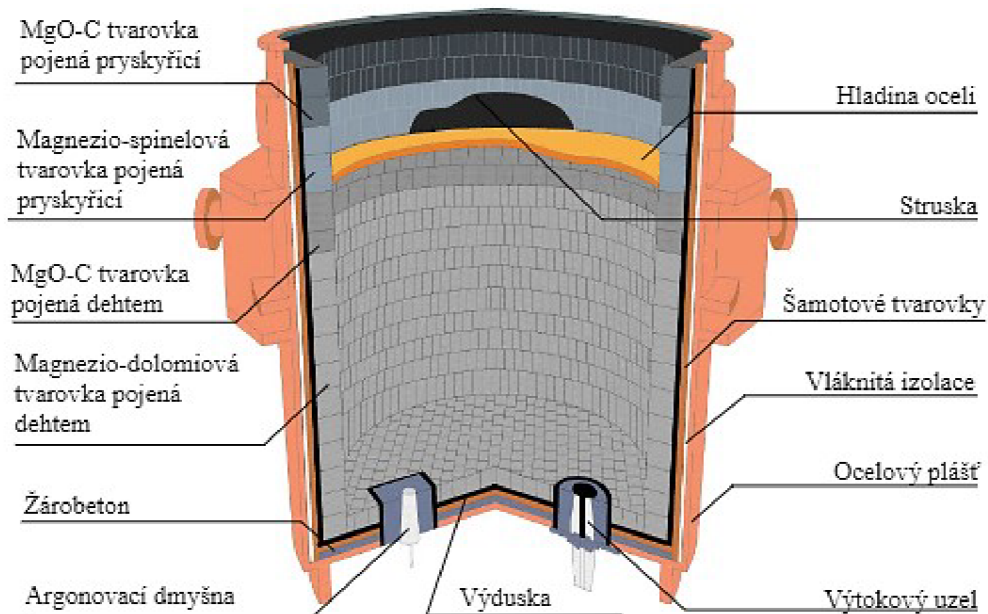
Obr. 18 Schéma vyzdívky lící pánve. [38]
