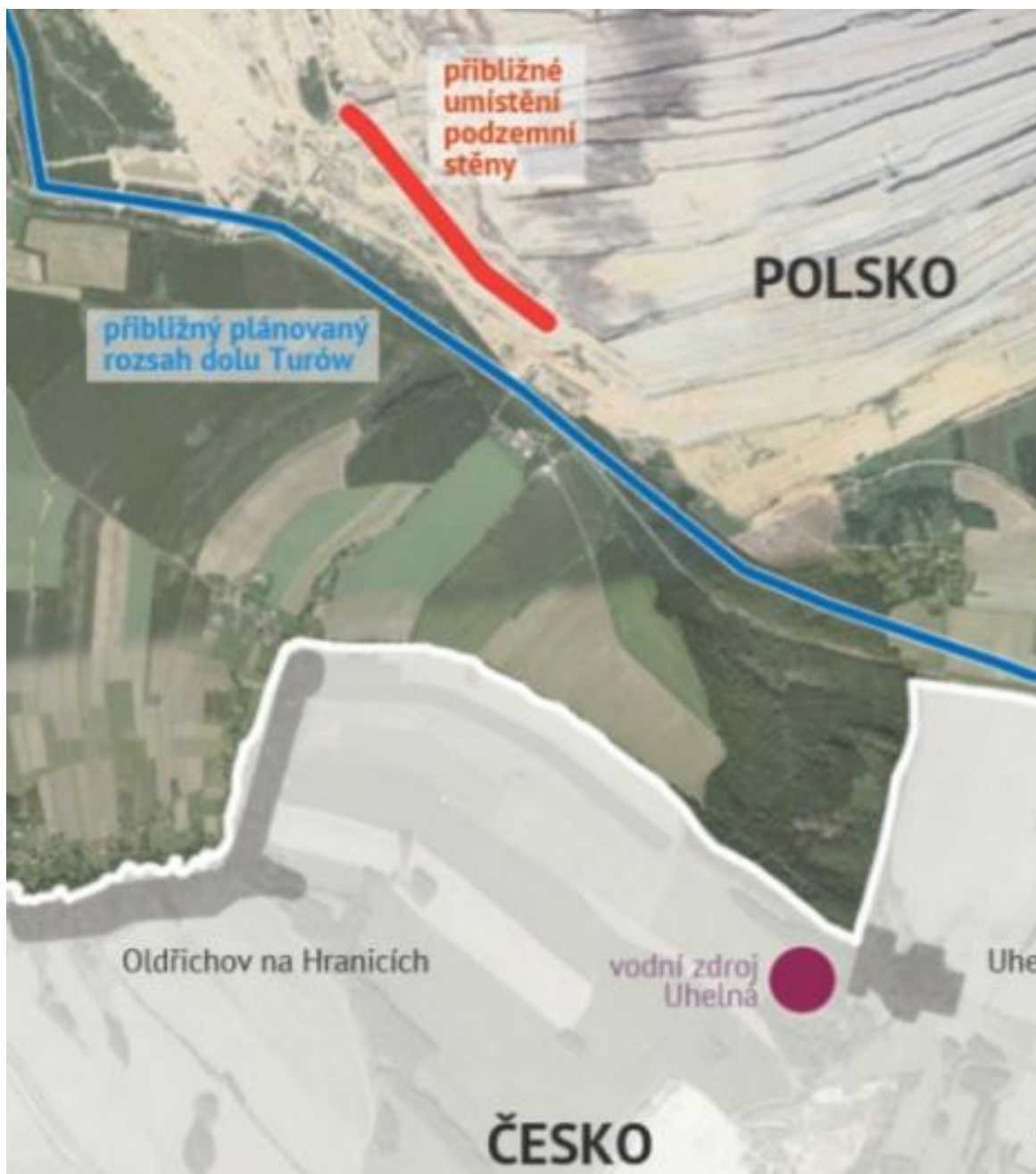
Obrázek 14 - Plánované rozšíření těžby (modrá linie) a označení ochranné těsnící stěny (červená linie).
