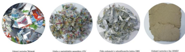
Obrázek 13: Postup recyklace nápojových kartonů [27]
