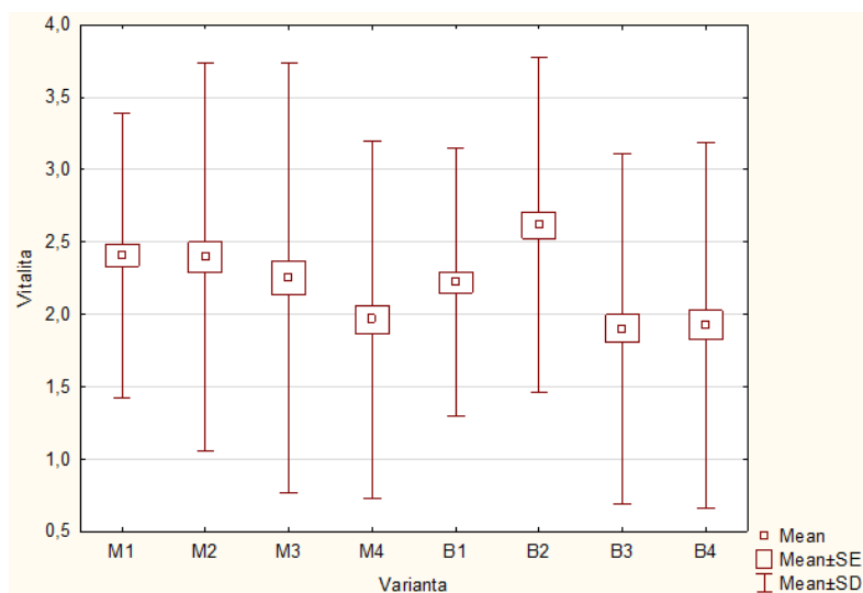
Obr. číslo 15: Porovnání vitality sazenic v roce 2019 podle jednotlivých variant (n= 1 296, p= 0)
