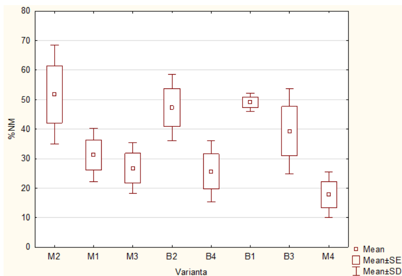
Obr. číslo 20: Porovnání procentuálního zastoupení neaktivních mykorhizních špiček u sazenic v roce 2021 podle jednotlivých variant (n= 24, p= 0,458)
