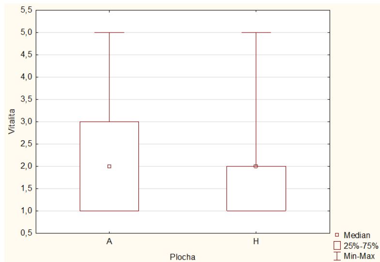
Obr. číslo 21: Porovnání vitality sazenic mezi plochou Apolenka (A) a Halže (H) v roce 2021
