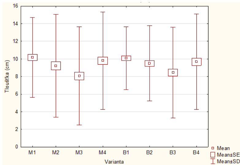
Obr. číslo 12: Porovnání tloušťky kořenového krčku sazenic v roce 2021 podle jednotlivých variant (n= 1 296, p = 0,0001)
