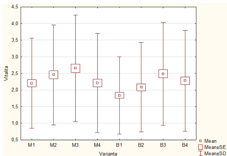
Obr. číslo 14: Porovnání vitality sazenic v roce 2021 podle jednotlivých variant (n= 1 296, p= 0)
