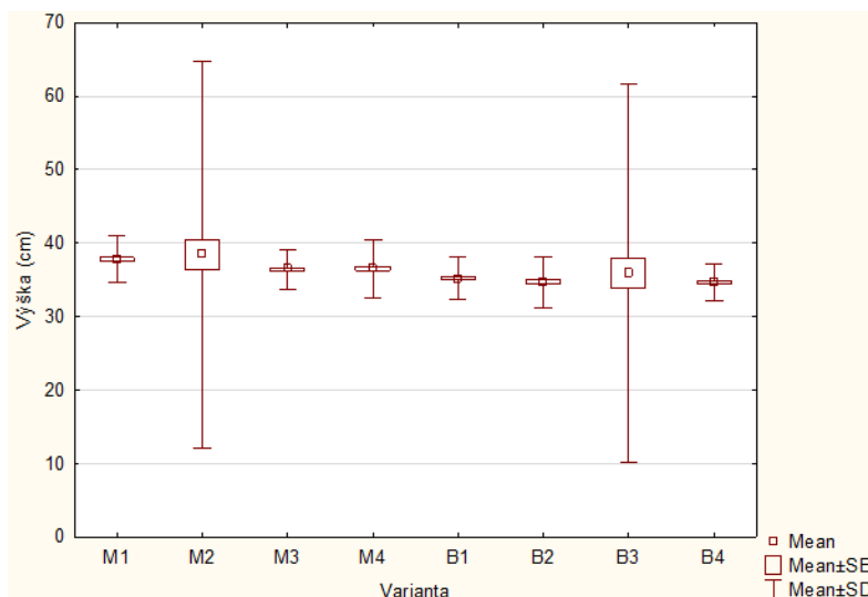
Obr. číslo 11: Porovnání výšky sazenice v roce 2019 podle jednotlivých variant (n= 1 296, p= 0)
