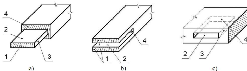
Obrázek 16. Čepované spoje
