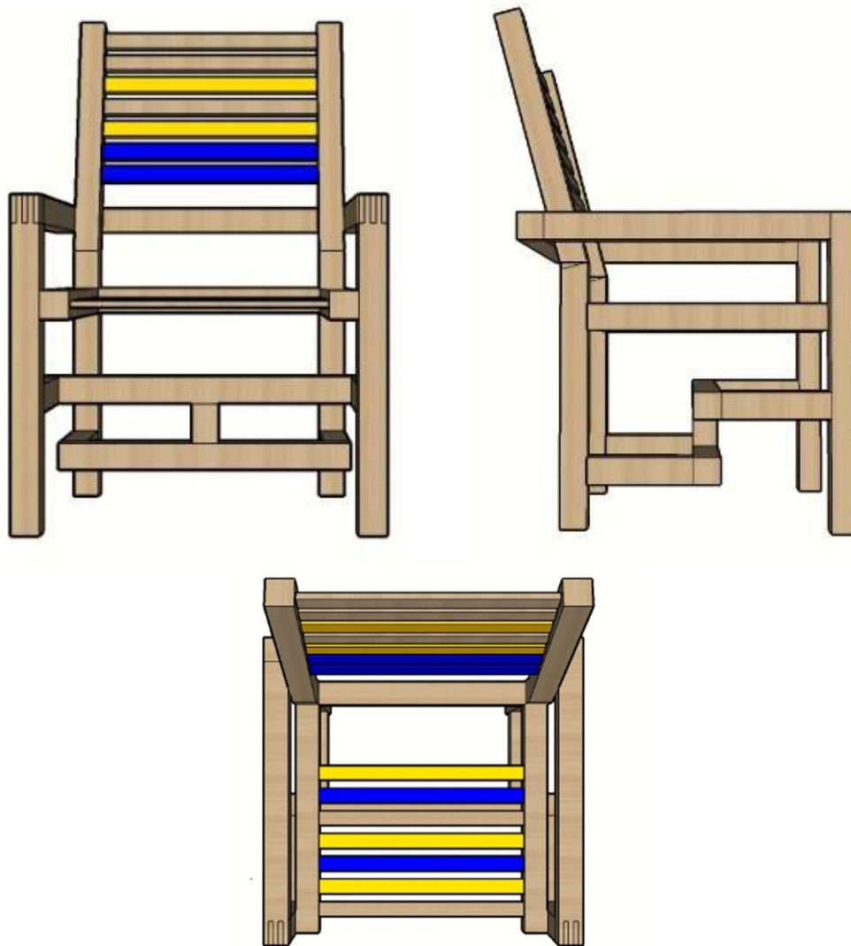
Obrázek 23. Návrh sedadla verze 5 - nárýsný, bokorysný a půdorysný pohled
