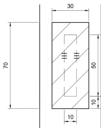
Obrázek 42. Nárysny řez spojení sedací části s bočnicí
