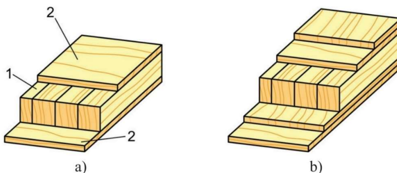
Obrázek 13. Vrstvy laťovek
