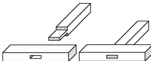
Obrázek 17. Čep a dlab s hranatým průběžným čepem
