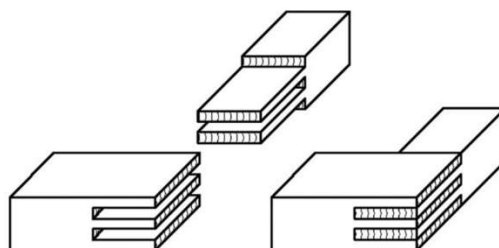
Obrázek 18. Rohový dvojitý čep a rozpor
