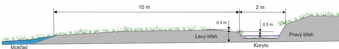
Obrázek č. 27: příčný profil nového koryta a tvar břehu (Jiří Václavek, 2022).
