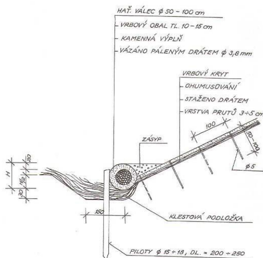
Obrázek č. 6 Usměrnující a stabilizační objekt haťošterkový válec (Šlezinger, 2010).
