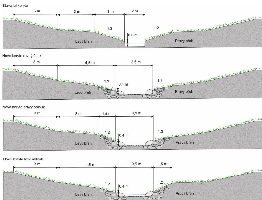
Obrázek č. 37: původní profil a návrh příčných profilů všech úseků koryta (Jiří Václavek, 2022).
