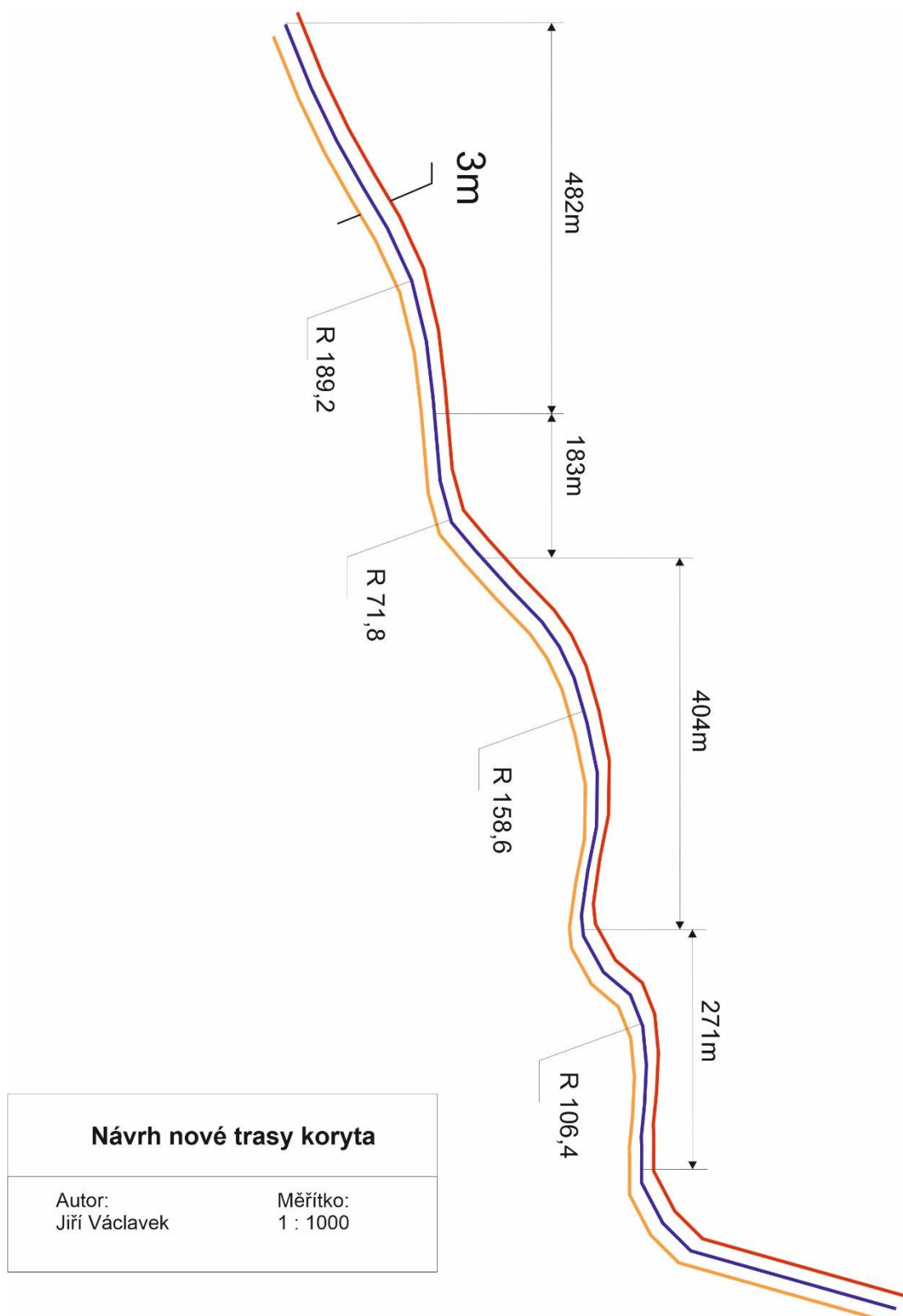
Obrázek č. 36: návrh kynety nového toku (Jiří Václavek, 2022).
