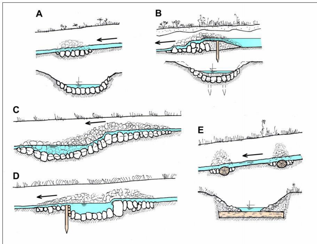
Obrázek č. 7 A – kamenitý práh ve dně, B - skluzový stupeň z kameniva a drnu C - skluzový stupeň s tůň z kameniva D - nízký stupeň s tůň z kameniva, s pomocnou stabilizační dřevnou kulatinou E – klády ve dně (Just et al., 2005)
