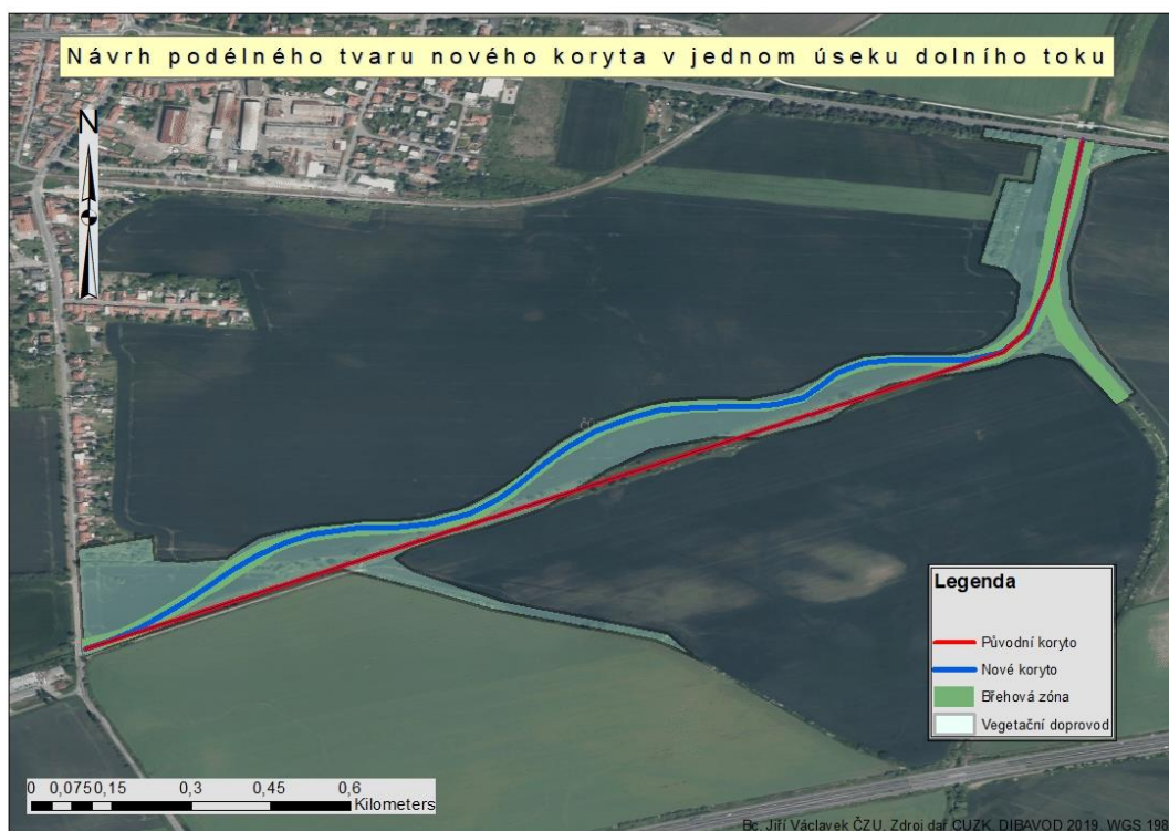
Obrázek č. 34: návrh podélného tvaru nového koryta třetího úseku dolního toku (Jiří Václavek, 2022).
