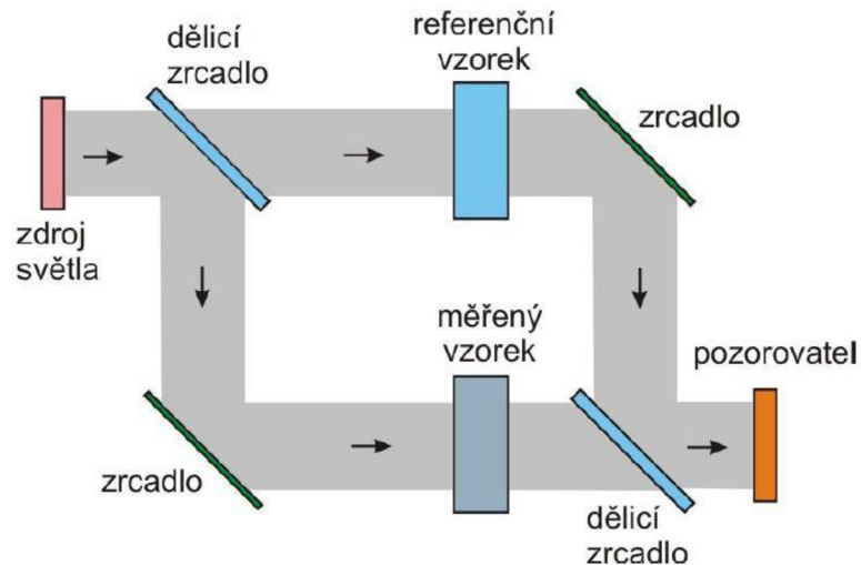
Obr. 6 Schéma Machova-Zehnderova interferometru [13].
