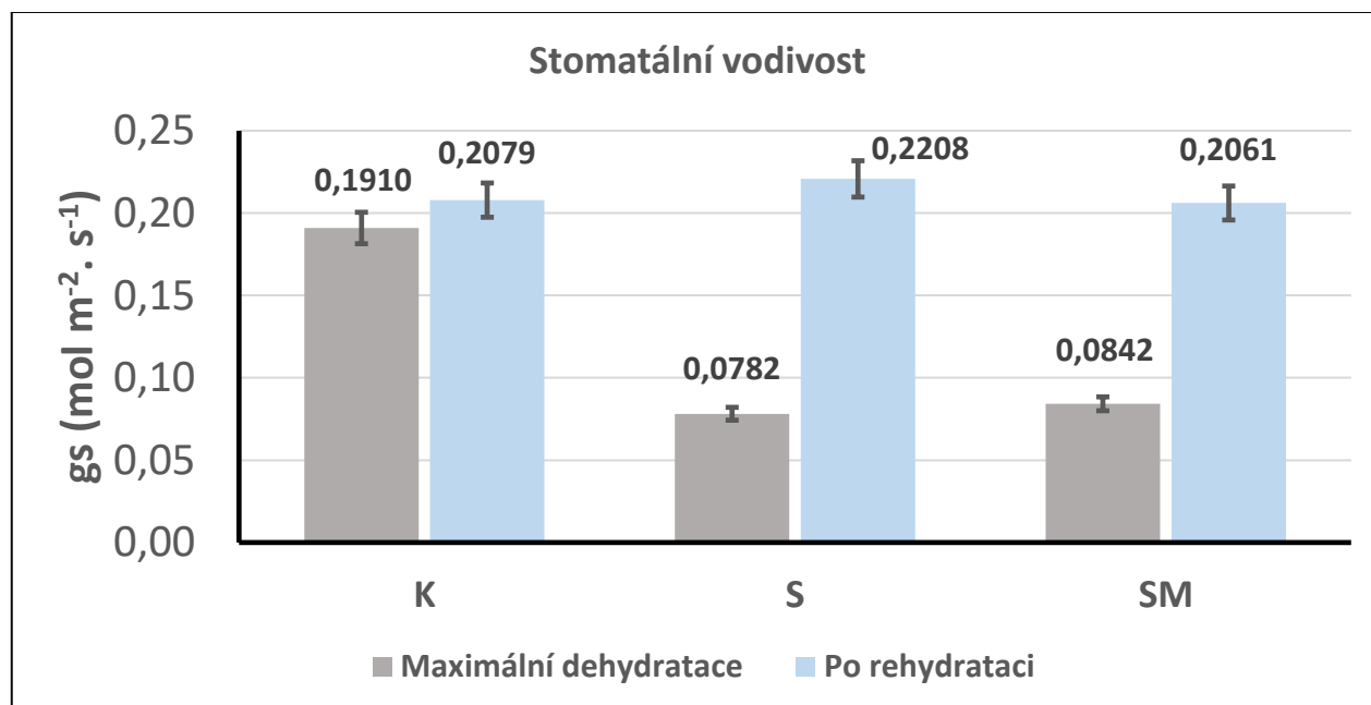
Obr. 3: Stomatální vodivost sledovaných variant rostlin ( g_s ; \text{mol m}^{-2} \text{s}^{-1} ): K – kontrola, v. S – stresovaná varianta bez aplikace melatoninu, v. SM – stresovaná varianta s aplikací melatoninu
