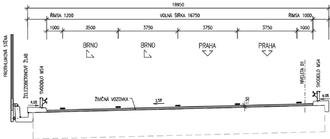
Obrázek 1 – Mostní svršek levého mostu ve směru Praha
