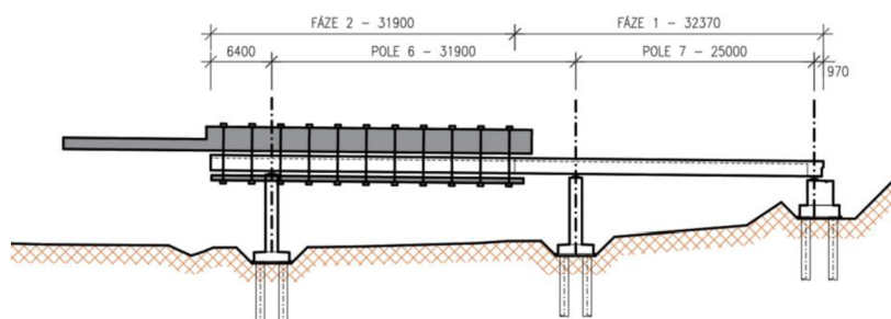
Obrázek 19 - Schéma výstavby druhého pole
