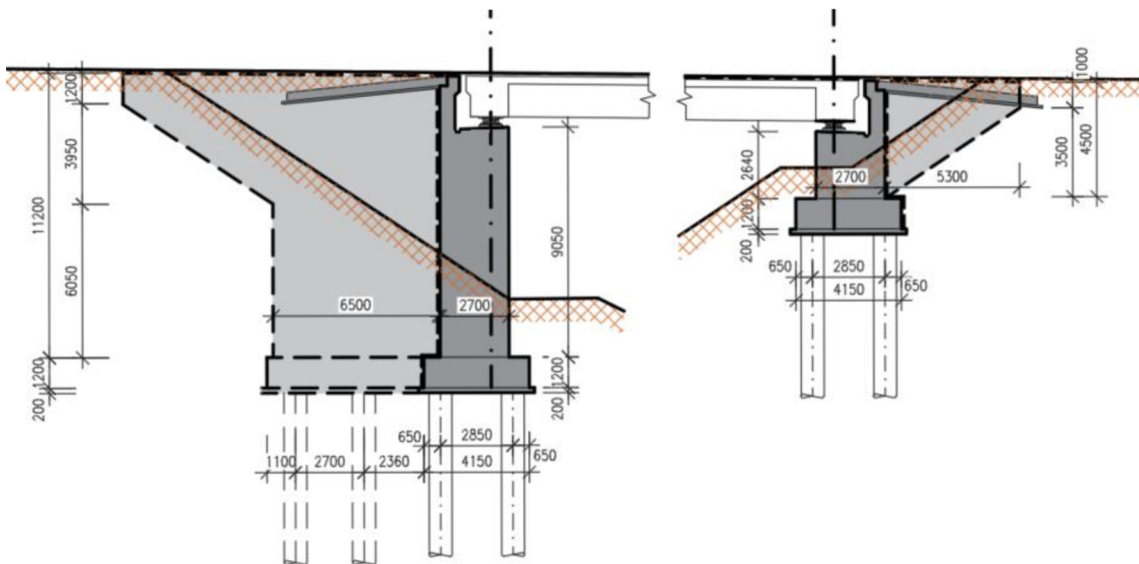
Obrázek 13 - Schéma krajních opěr a křídel
