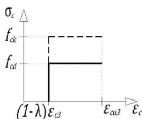
Obrázek 42 – Obdélníkový pracovní diagram betonu
