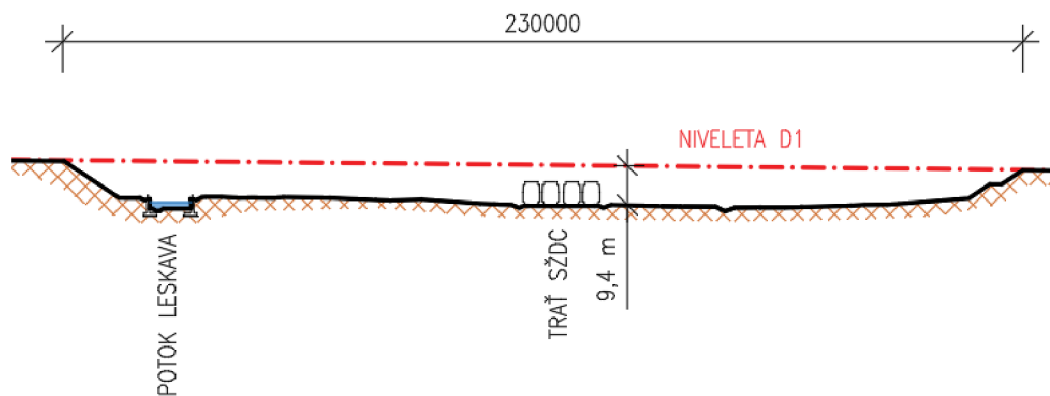
Obrázek 3 - Podélný řez terénem s niveletou komunikace
