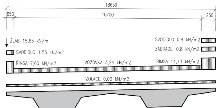
Obrázek 37 - Schéma příčného řezu s vykreslením zatížení od jednotlivých částí mostního svršku
