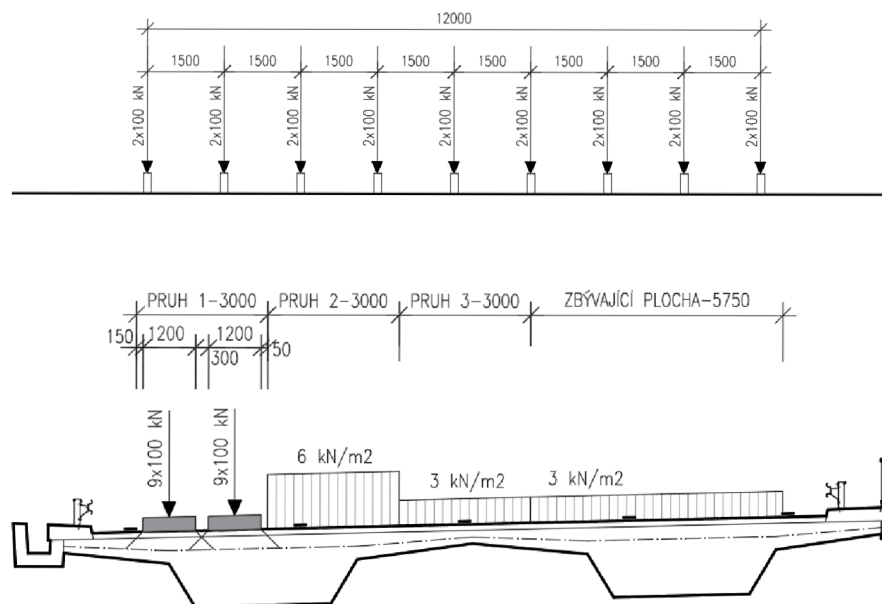
Obrázek 40 - LM3 - 1800/200, poloha zatížení v příčném a podélném směru
