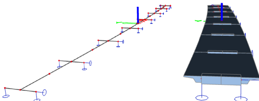
Obrázek 32 - Prutový model
