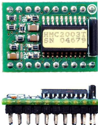
Obr. 2.13. Snímač HMC2003 [15]
