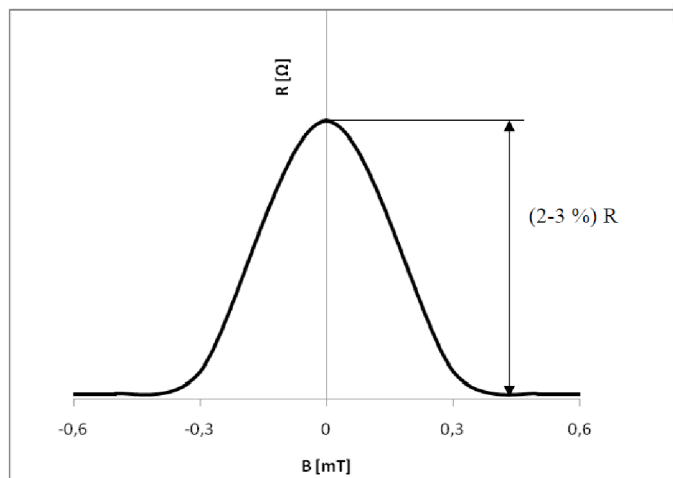
Obr. 2.3 Závislost odporu na velikosti magnetického pole [2]
