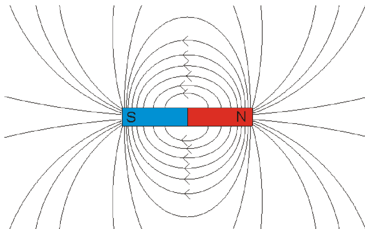
Obr. 2.1. Magnetické indukční čáry tyčového magnetu [3]
