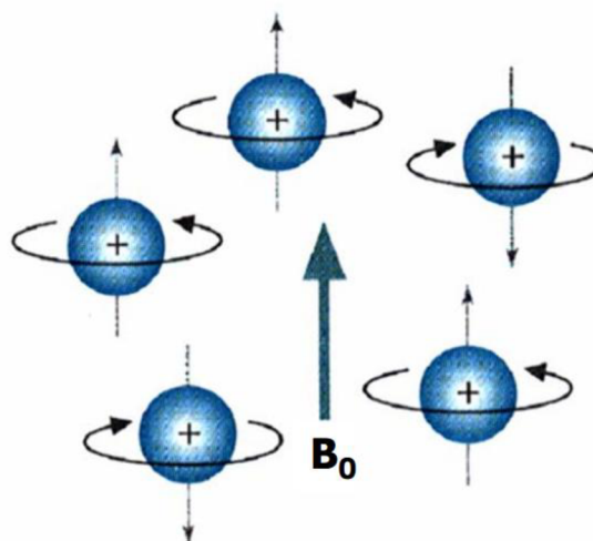
Obr. 2.10. Protony ve vnějším magnetickém poli [13]
