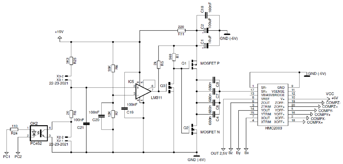
Schéma části: resetovací obvod
