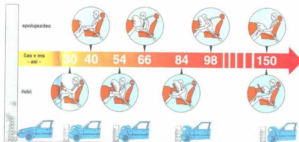
Obrázek 1: Průběh nafukování airbagu
