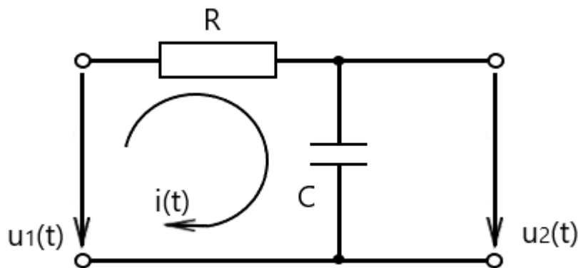
Obrázek 1.1.4: Schéma zapojení RC článku
