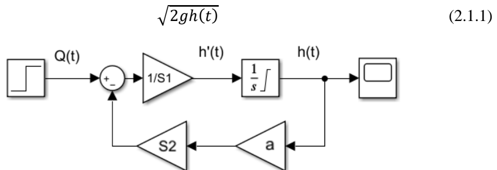
Obrázek 2.1.2: Schéma parametrizovaného systému MATLAB Simulink
