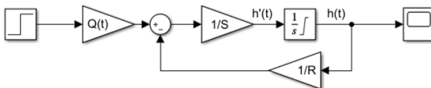
Obrázek 2.1.4: Schéma linearizovaného hydraulického systému
