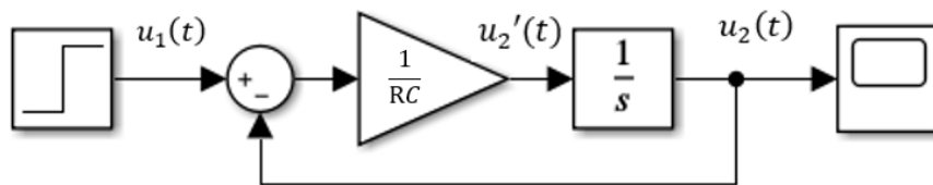
Obrázek 2.1.9: Schéma linearizovaného RC článku
