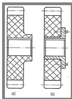
Obr. 6-2 Úpravy pro snížení tlaku v drážce pro pero [1]
