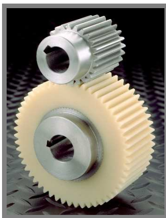
Obr. 2-1 Nastříknutý věnec na kovový kotouč [9]
