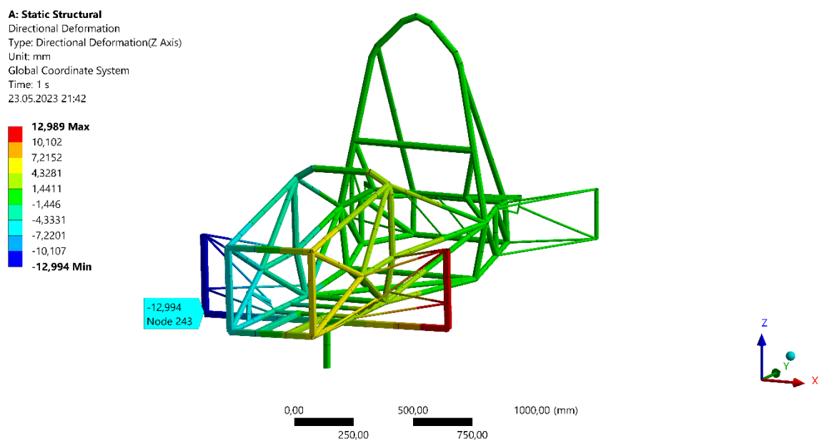
Obrázek 23: Výsledné posunutí přední nápravy rámu formule 3. generace
