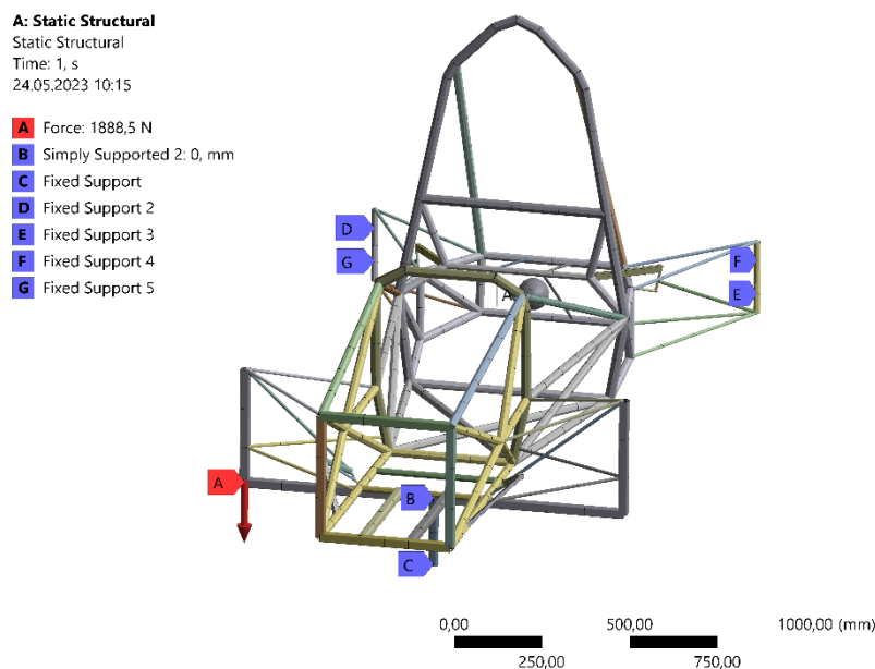
Obrázek 21: Zobrazení okrajových podmínek na MKP modelu rámu formule 4. generace
