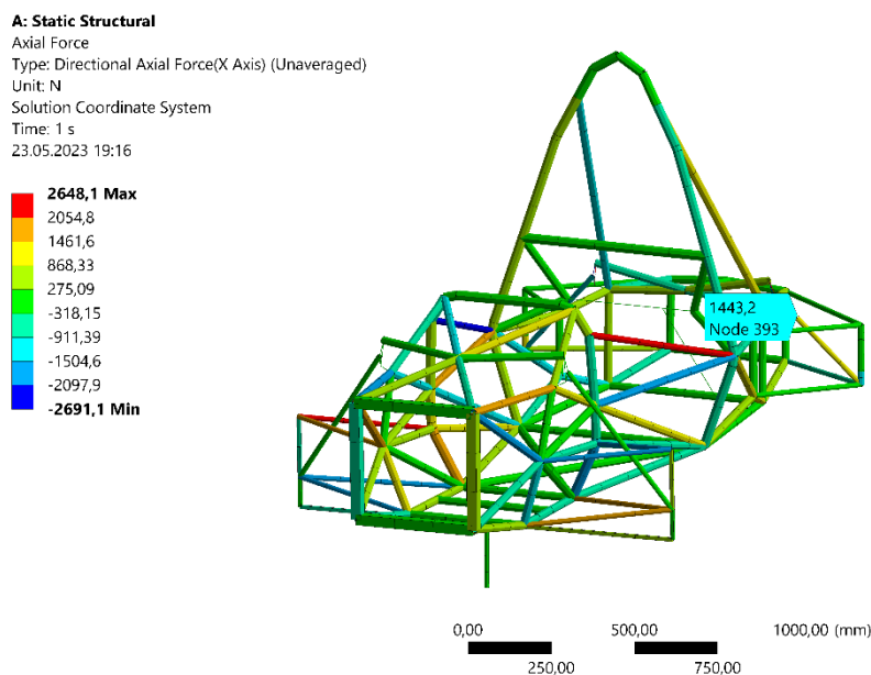
Obrázek 16: Zobrazení výsledné axiální síly v jednotlivých profilech u rámu formule 4. generace
