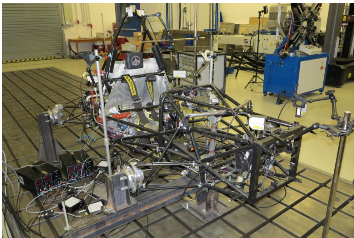
Obrázek 9: Rák 4. generace připravený na měření torzní tuhosti
