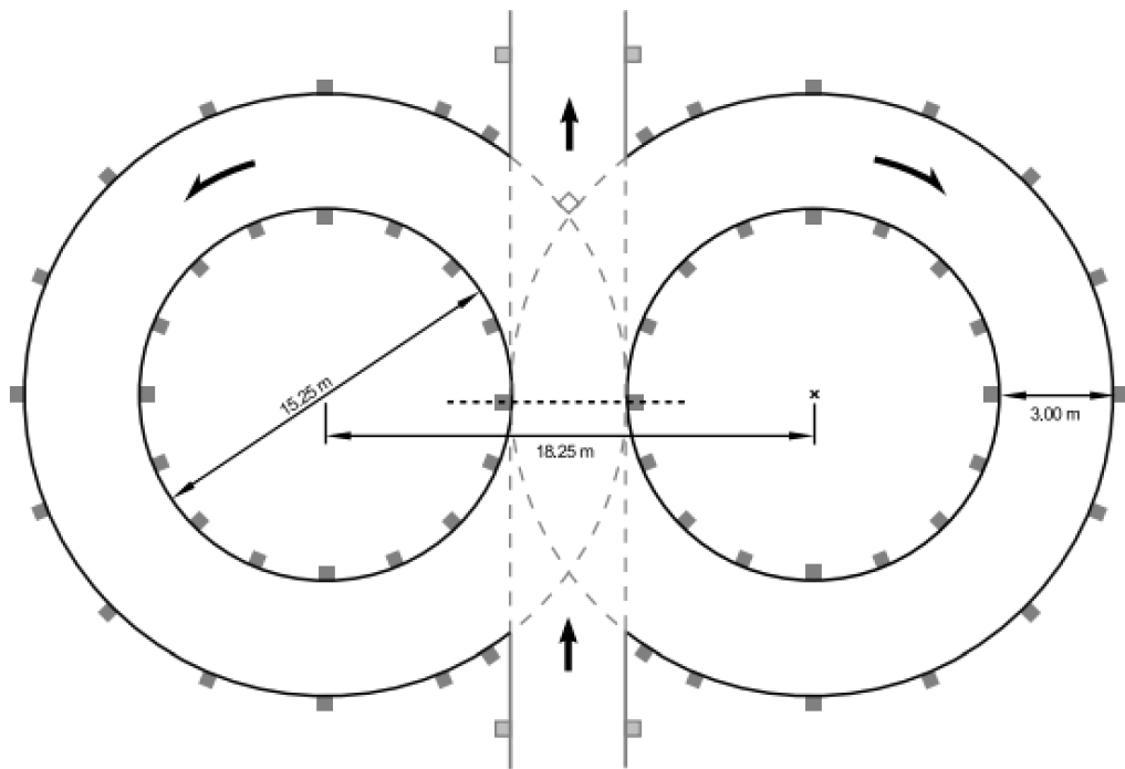
Obrázek 2: Trať disciplíny Skid Pad [13]
