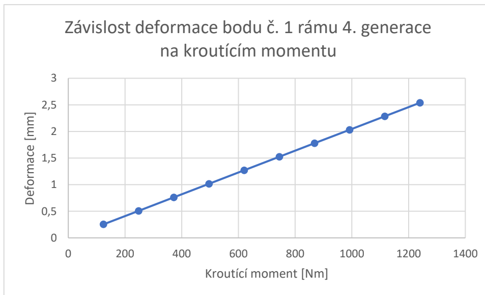
Obrázek 26: Hodnoty posunutí bodu č. 1 rámu formule 4. generace při rostoucím zatěžování
