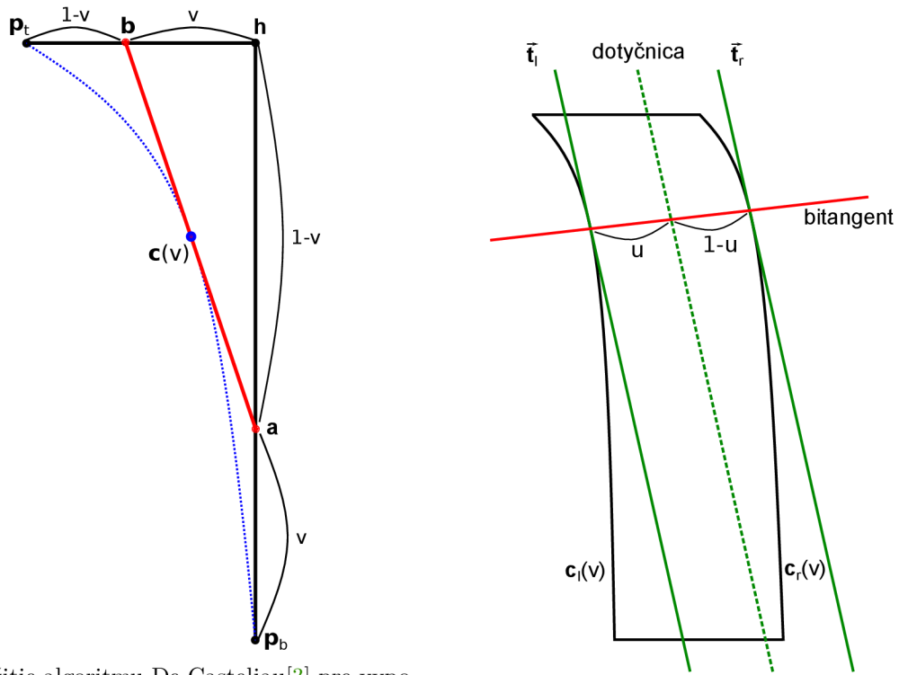
(b) Ukážka výpočtu dotyčnice a bitangentu stebra trávy.
