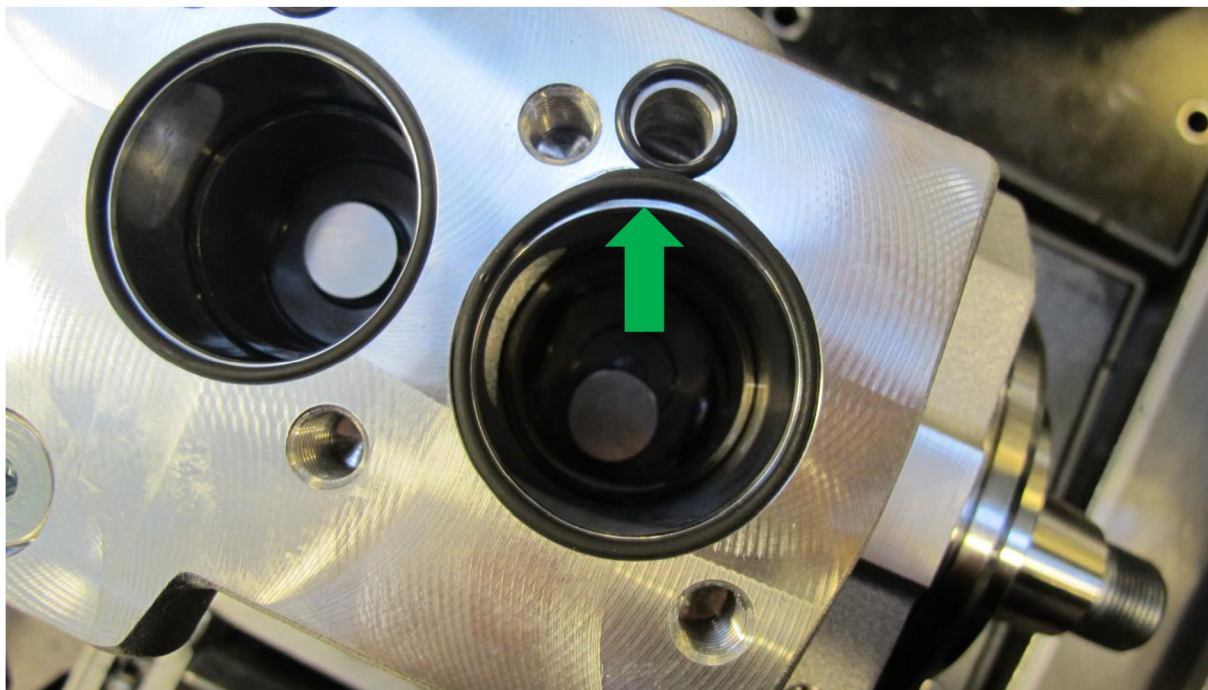
Obrázek 16: Poškození o-kroužku [1]
