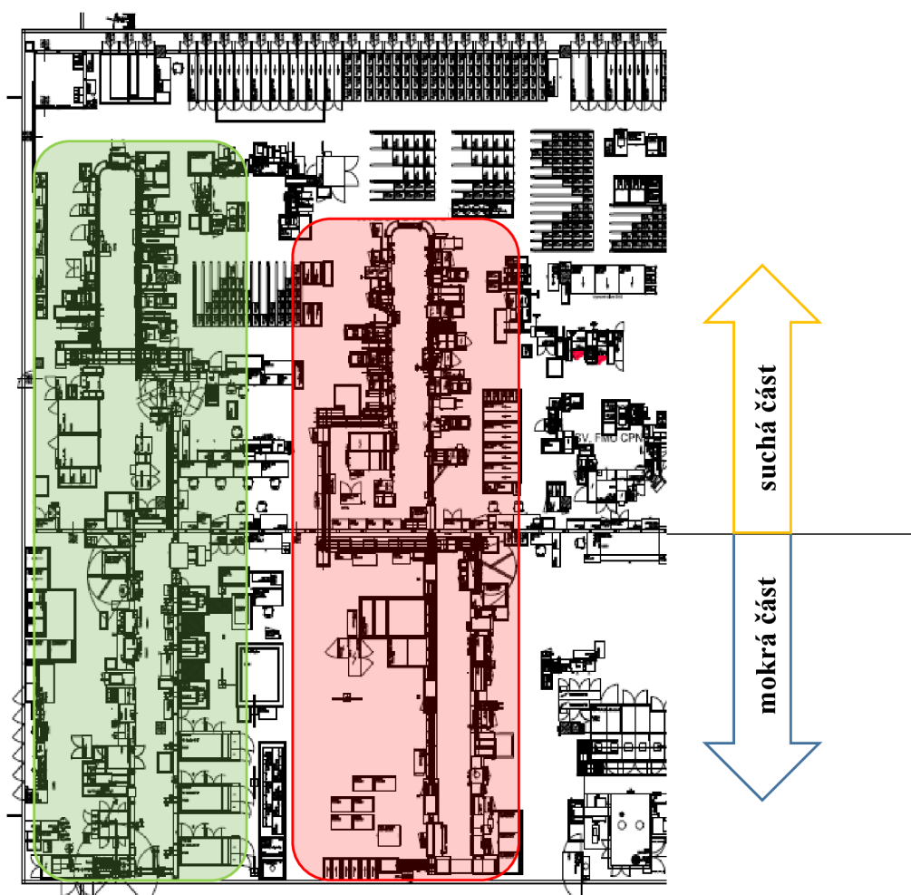
Obrázek 6: Montážní linky čerpadel 1 (zeleně) a 2 (červeně) [1]
