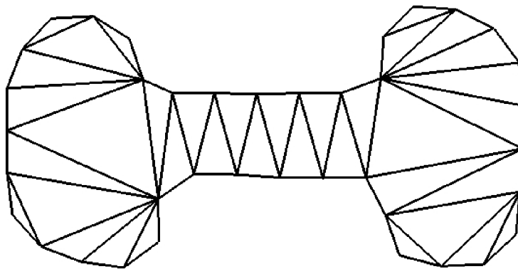
Obrázek 4.6: Síť bez externích trojúhelníků
