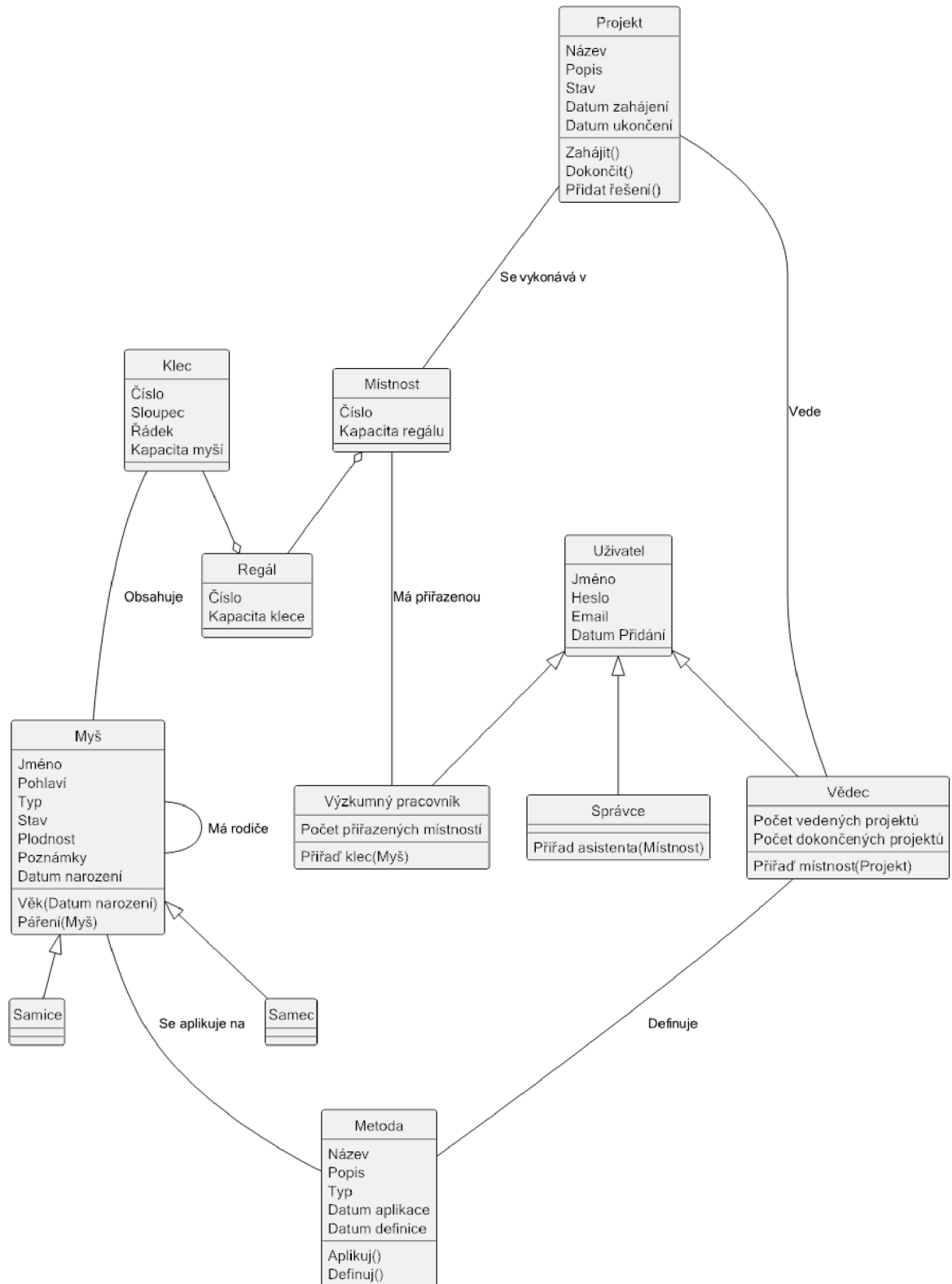
Obrázek č. 27: Class diagram [autor]
