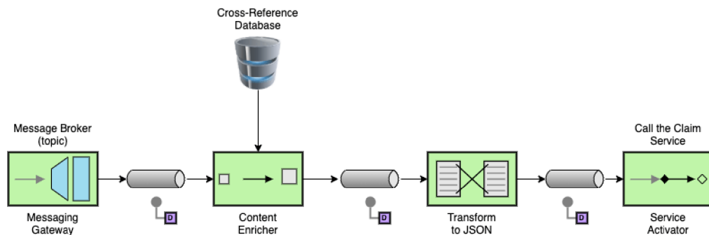
Obrázek č. 9: Pipeline architektura. [28]
