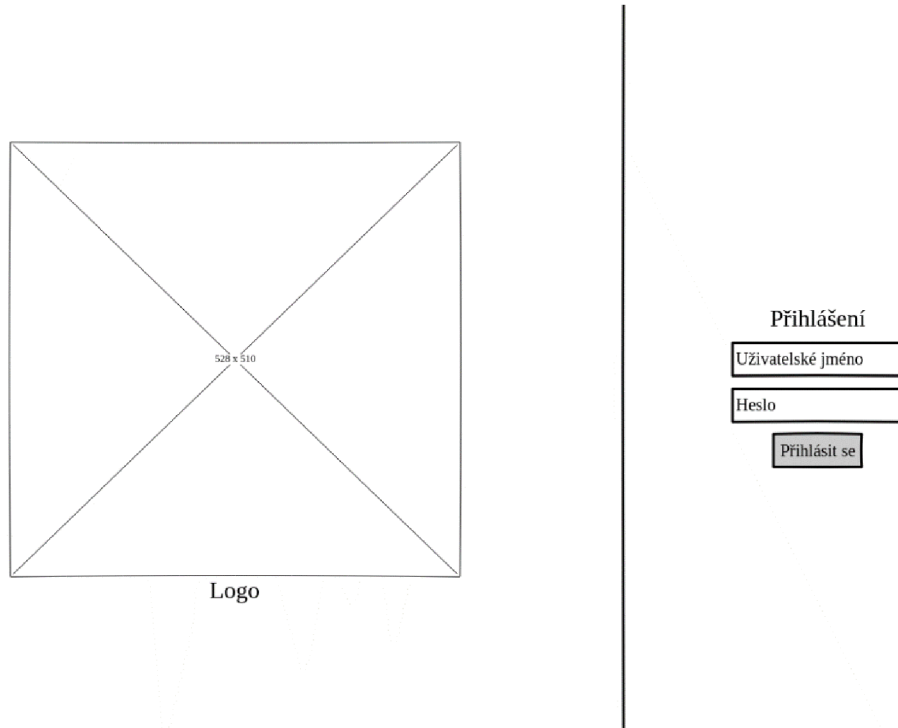
Obrázek č. 32: Wireframe přihlášení [autor]
