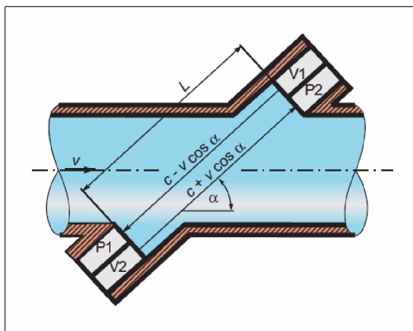
Obrázek 4: Přímý ultrazvukový průtokoměr-princip[4]
