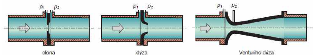
Obrázek 1: Průřezové průtokoměry [3]
