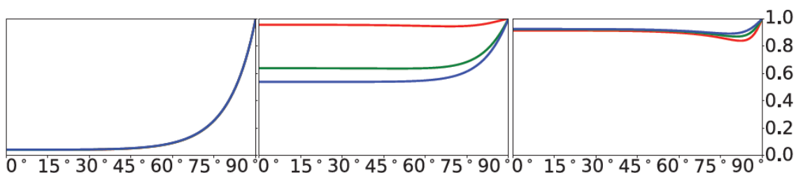
Obr. 1 Příklady hodnot Fresnelovy funkce (zleva): sklo, měď, hliník. Převzato z Real-Time Rendering [4].
