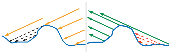
Obr. 8 Vizualizace zastínění (nalevo) a maskování (napravo). Převzato z Real-Time Rendering [4].
