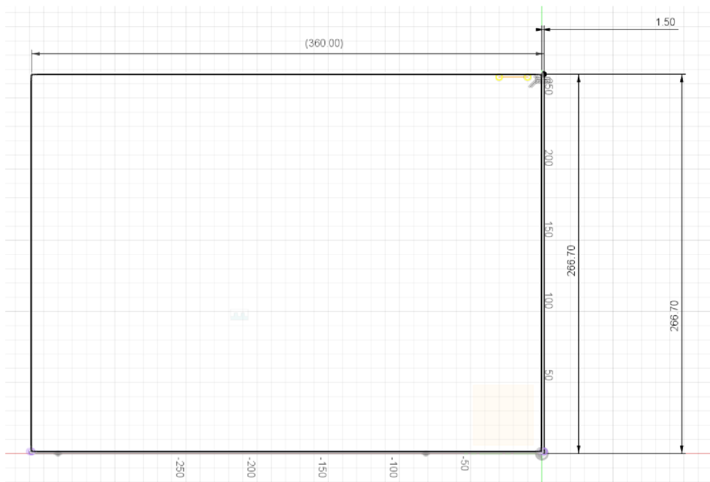
Obr. D.2: Parametry bočnice skříně.
