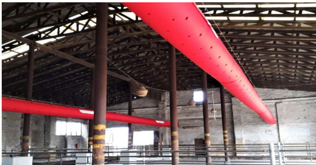
Obrázek 3.3: Tubusové větrání (Agrico.cz, 2008)
