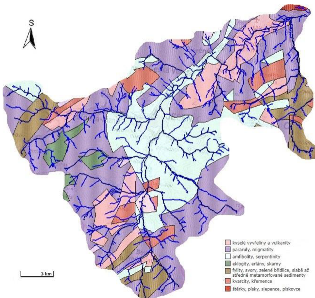
Obr. 15 – Horninové složení na toku Bělá dle Demka
