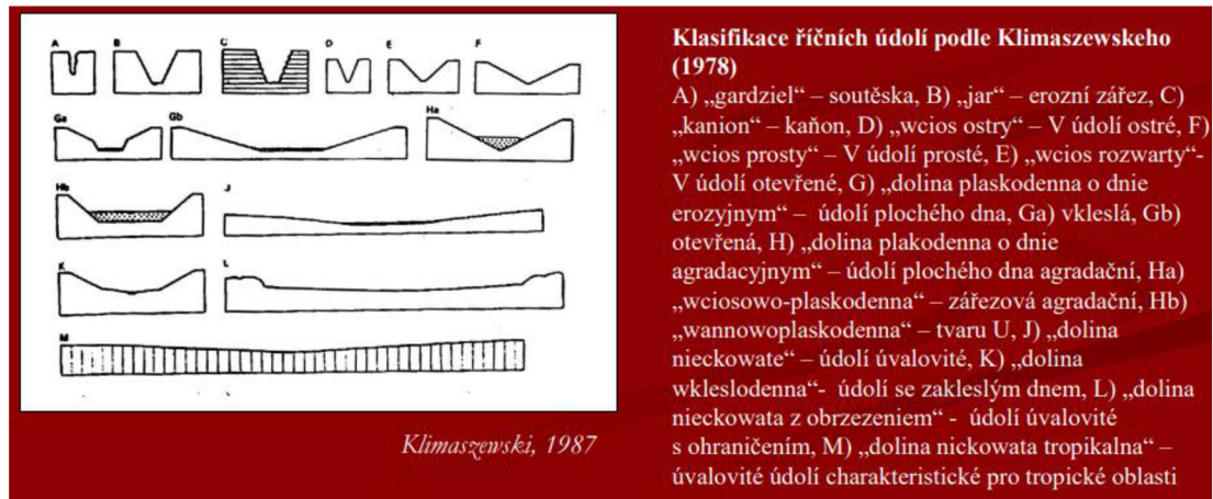
Obr. 5 – Klasifikace říčních údolí dle Klimaszewského
