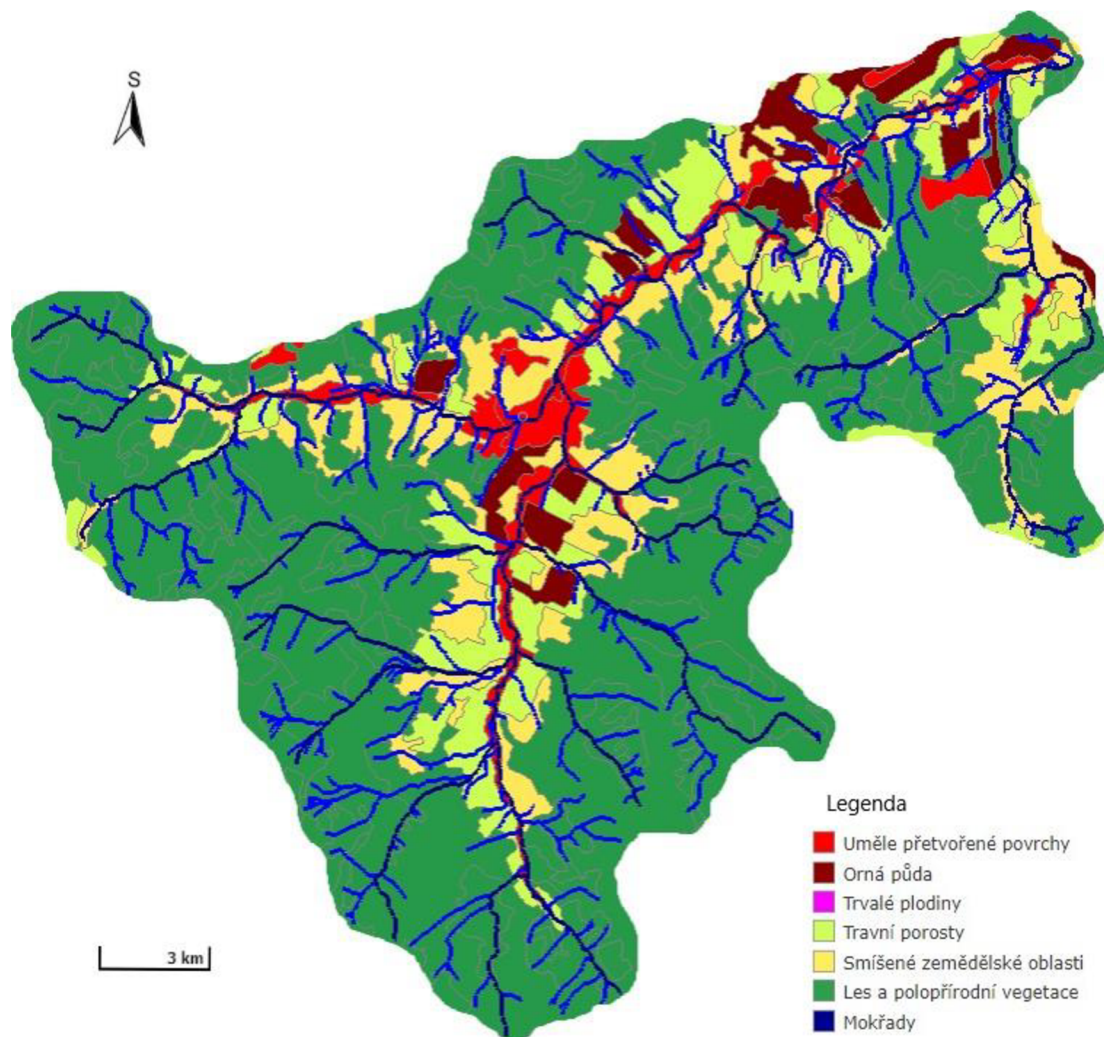
Obr. 11 – Krajinný pokryv povodí Bělé
