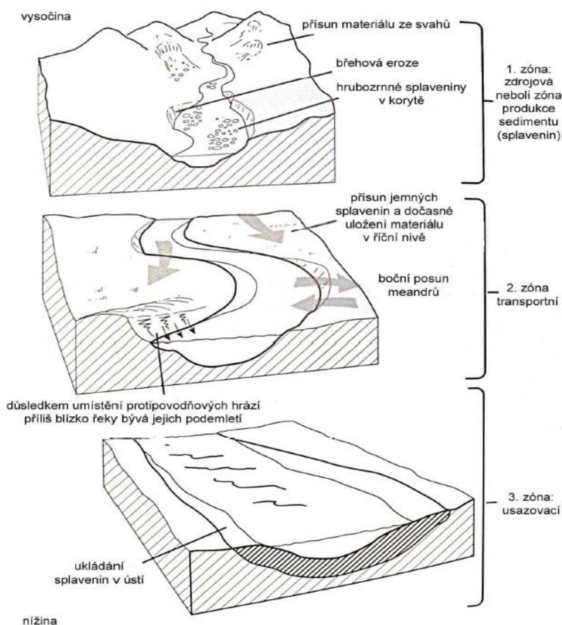
Obr. 3 – Zonální morfologické dělení
