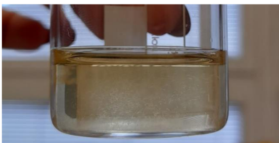
Obrázek 24: Sedimentovaná hád'átka.
