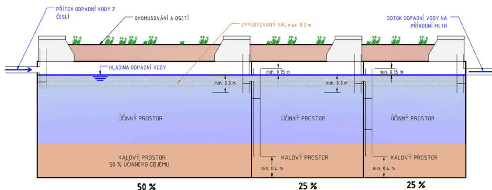
Obr. č. 14: Prostorové uspořádání anaerobního separátoru
