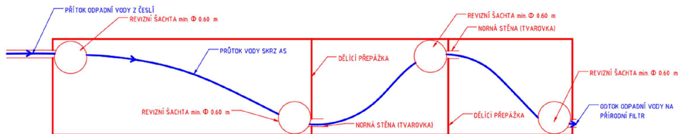
PŮDORYS ANAEROBNÍHO SEPARÁTORU S NAZNAČENÍM PROUDĚNÍ VODY
