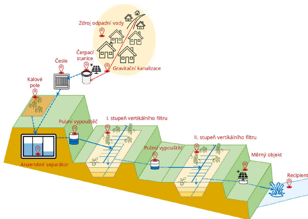
Obr. č. 22 Výškové uspořádání dvoustupňového vertikálního filtru
