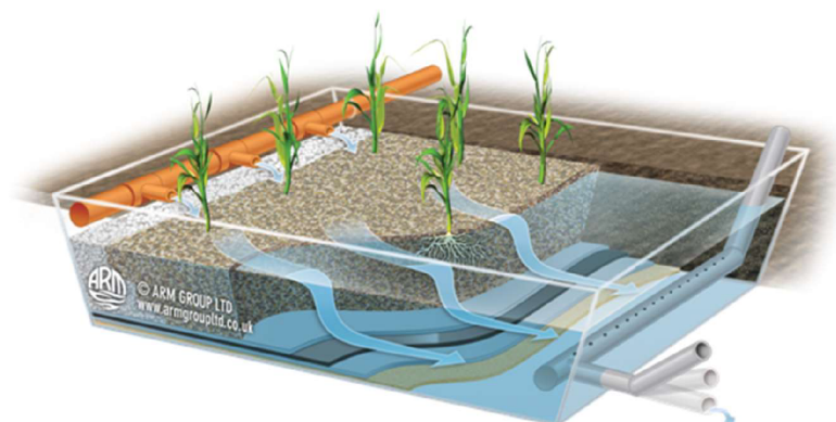
Obr. č. 18 Schéma horizontálního filtru převzato z („Global wetland technology“, n. d.)
