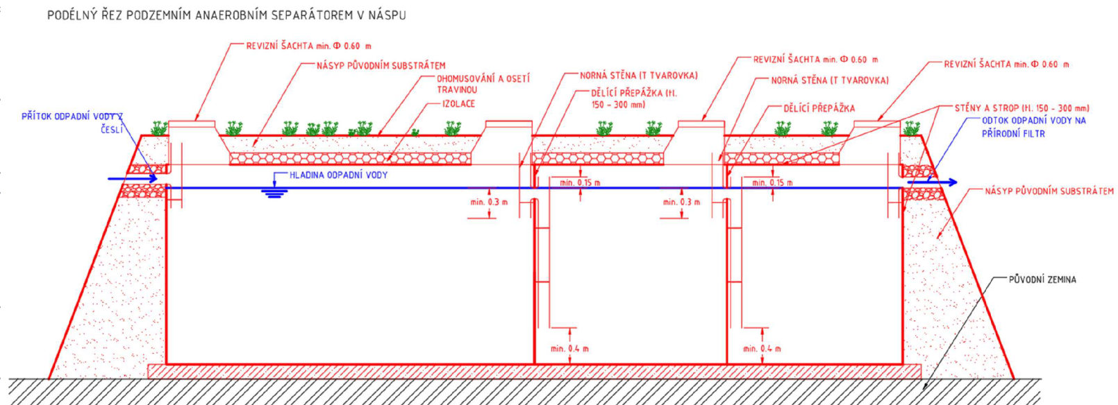
Obr. č. 44 Vzorový technický výkres anaerobního separátoru v náspu
