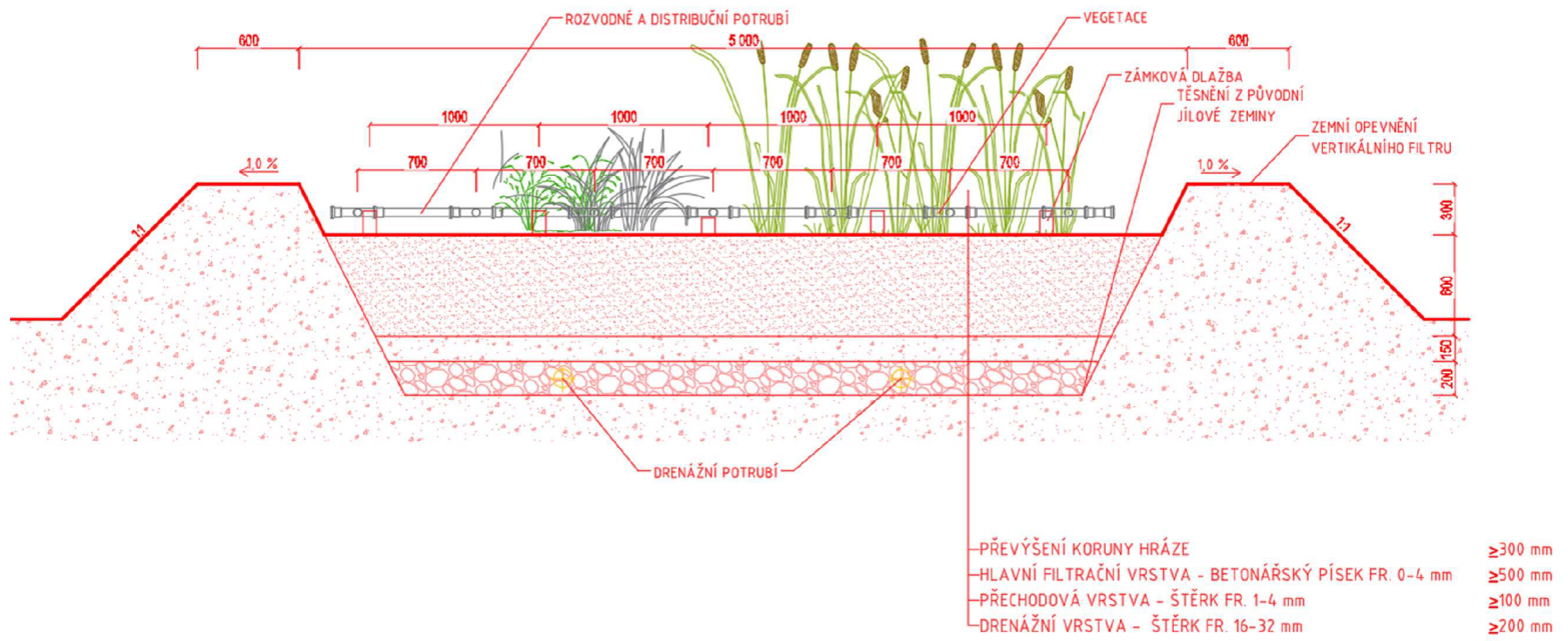
Obr. č. 46 Vzorový příčný řez II. stupněm vertikálního filtračního pole
