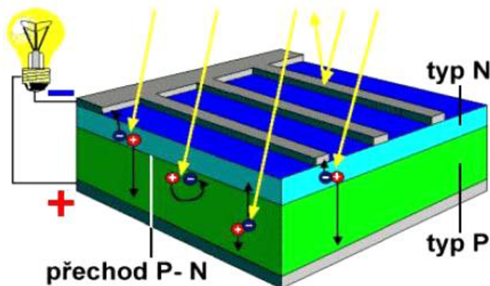
Obr. 1.2 Princip fotovoltaického článku [4]
