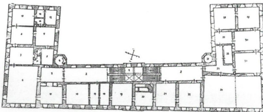
Obr. 106. Hradiště Mn. Zámek. Půdorys přízemku (nahore) a 1. patra (dole). Vue en plan du rez-de-chaussée et du 1er étage.
