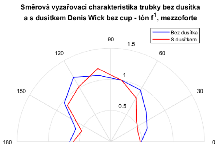
Graf 6.34: Směrová vyzářovací charakteristika trubky s rovným dusítkem Denis Wick
