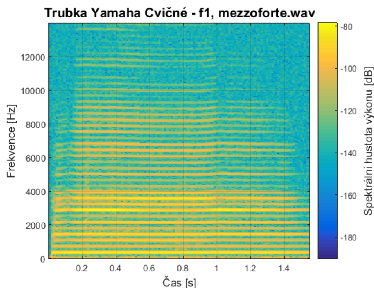
Graf 6.47: Spektrogram trubky s cvičným dusítkem
