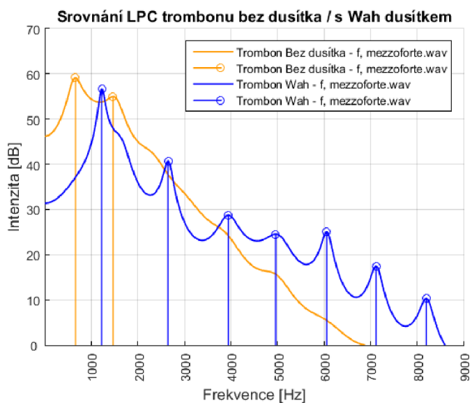
Graf 6.22: LPC trombonu s wah dusítkem
