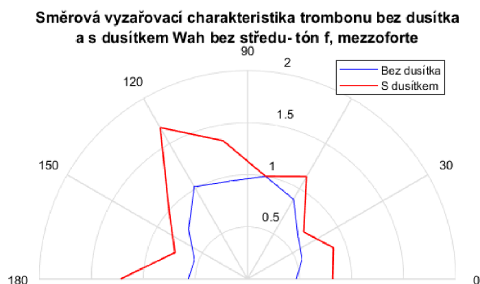
Graf 6.25: Směrová vyzářovací charakteristika trombonu s wah dusítkem bez středu
