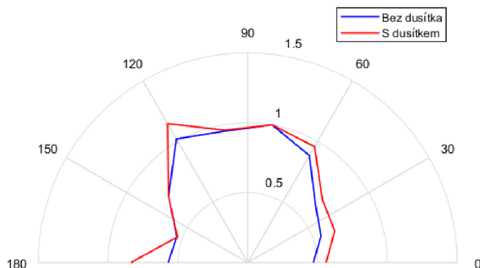
Graf 6.13: Směrová vyzářovací charakteristika trombonu s vatovým clamp dusítkem
