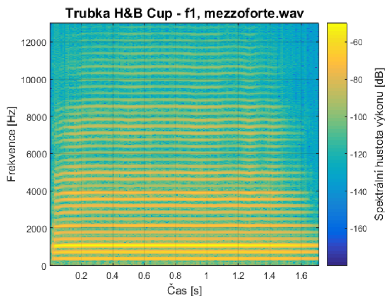
Graf 6.39: Spektrogram trubky s dusítkem cup Humes&Berg
