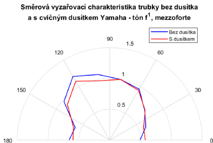
Graf 6.50: Směrová vyzařovací charakteristika trubky s cvičným dusítkem
