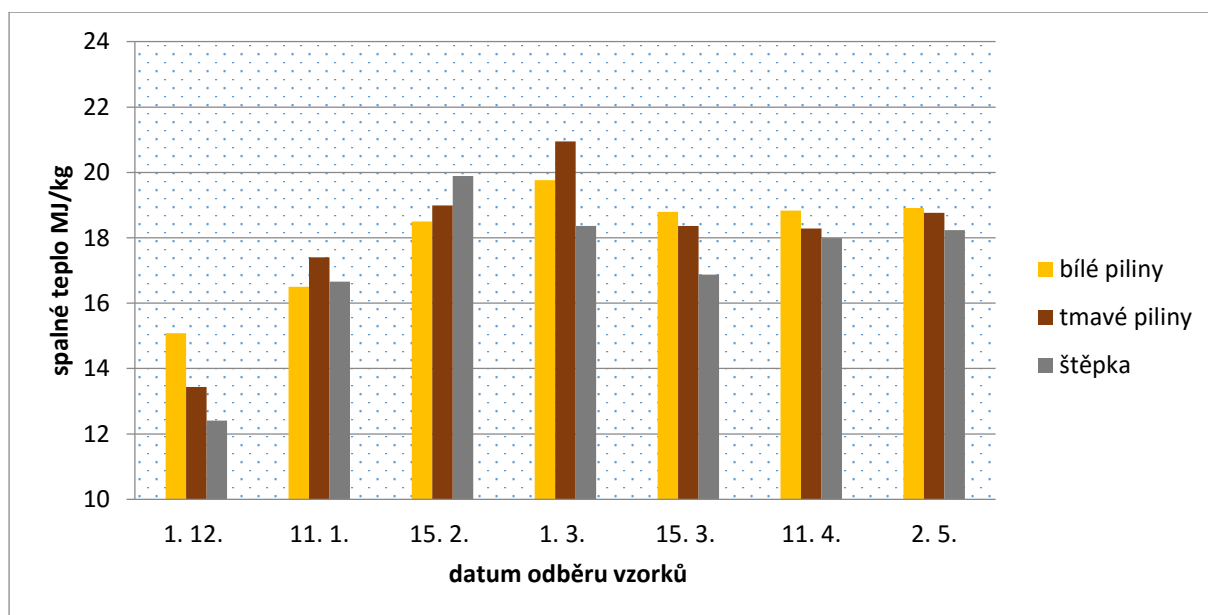
Graf 3 Naměřené hodnoty spalného tepla za měřený úsek
