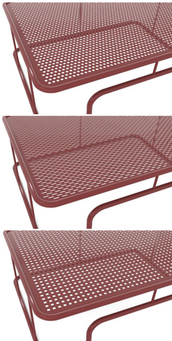
Obr. 23 Možnosti perforace
