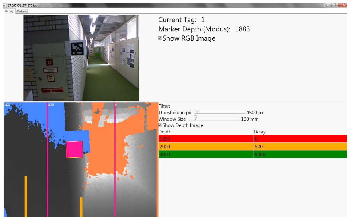
Obr. 3: Aplikace detekující značky.[5]
