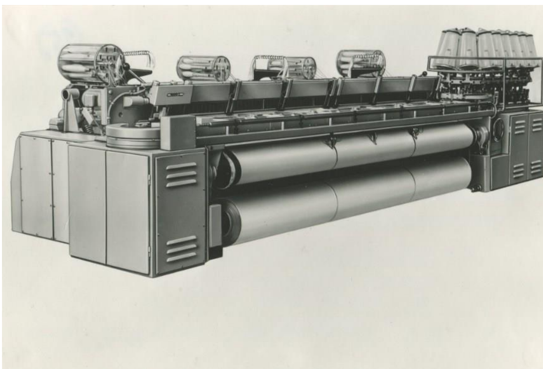
Obr. 8 - Tkací stroj Kontis (zdroj: Muzeum regionu Valašsko)
