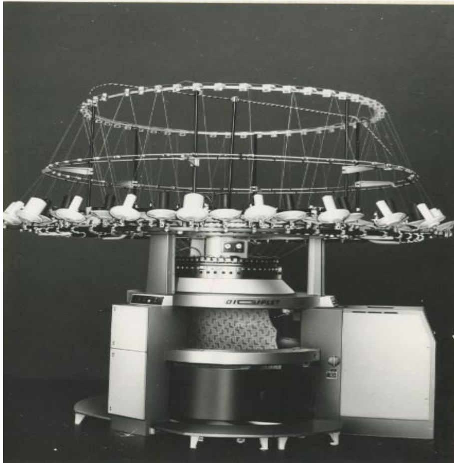
Obr. 11 - Pletací stroj Digiplot (zdroj: Muzeum regionu Valašsko)
