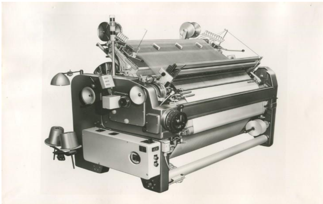
Obr. 5 - Vzduchový tryskový stav P 105 (zdroj: Muzeum regionu Valašsko)
