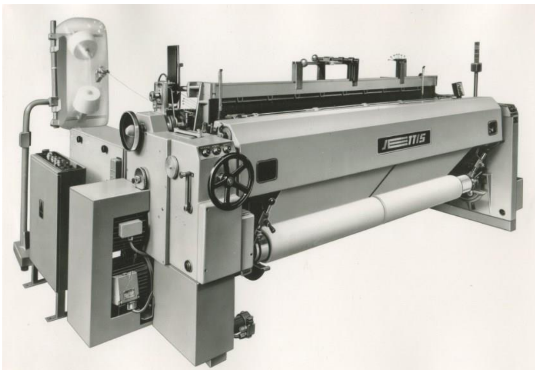
Obr. 7 - Tkací stroj Jettis (zdroj: Muzeum regionu Valašsko)
