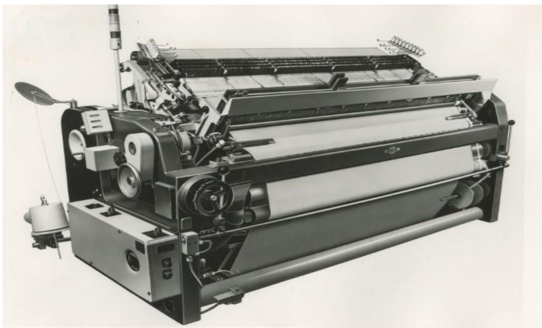
Obr. 6 - Vzduchový tryskový stav P 165 (zdroj: Muzeum regionu Valašsko)
