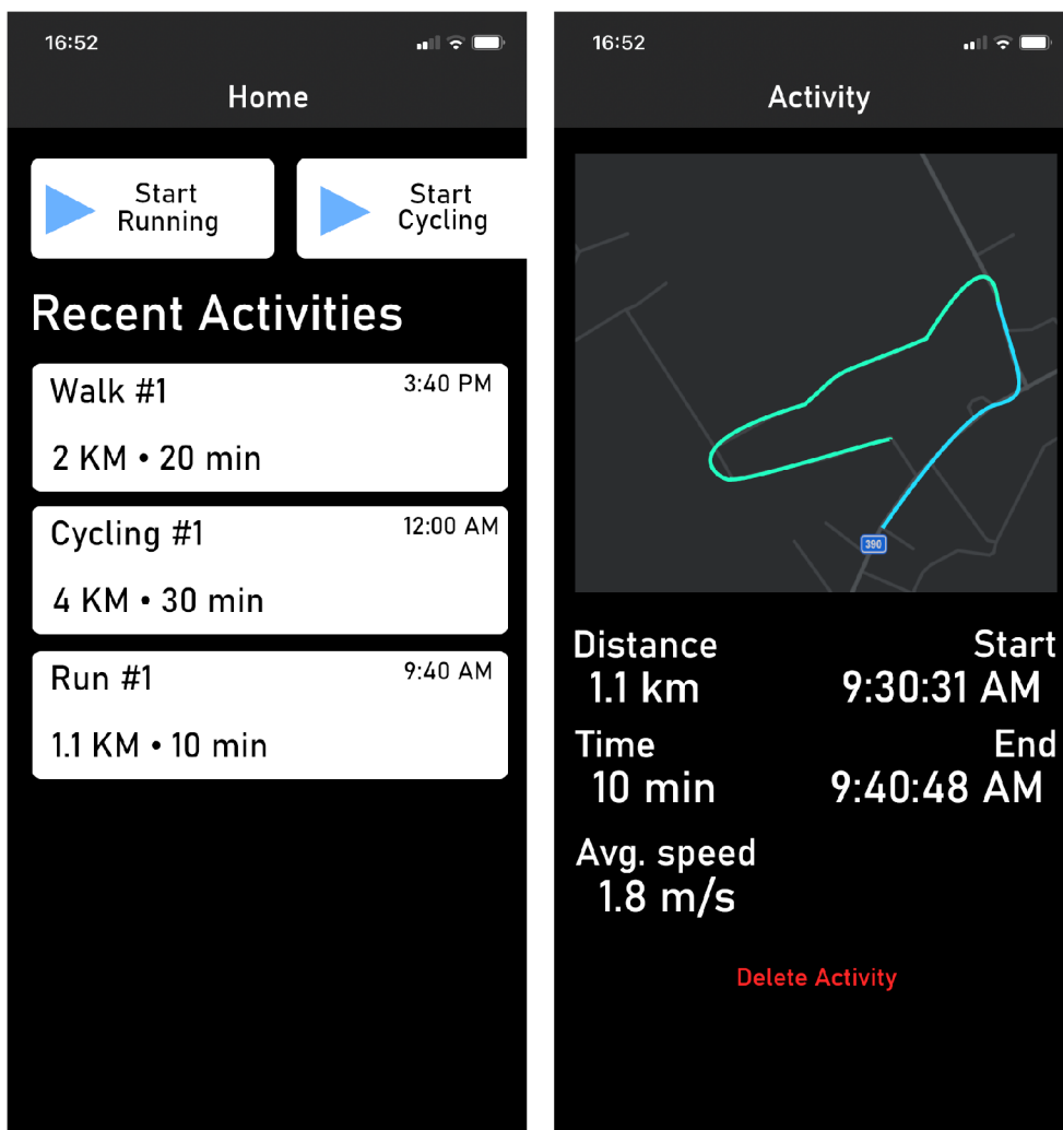
Obrázek 5.1: Návrh rozhraní mobilní aplikace
