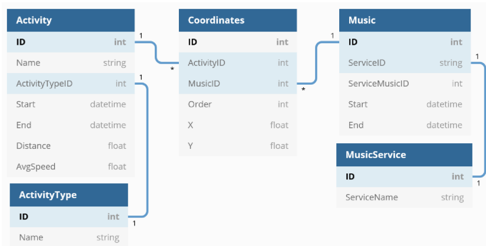
Obrázek 5.2: Digram entit
