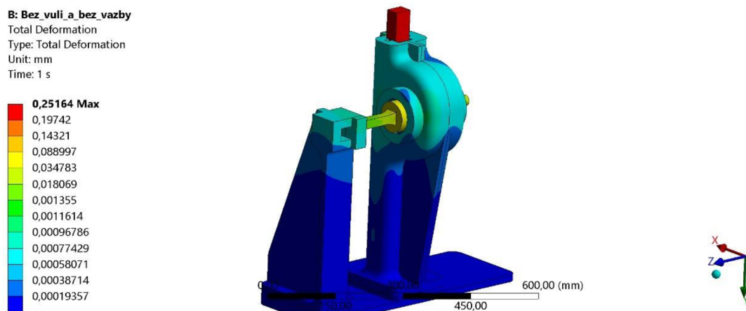
Obr. 5-12 Deformace přípravku druhé varianty (zvětšen rozsah barev pro lepší přehlednost)
