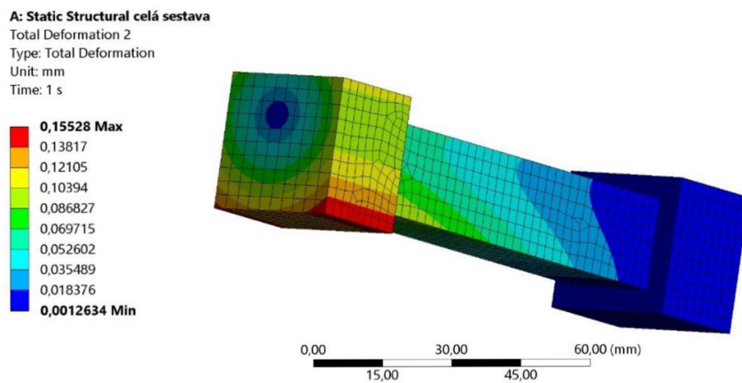
Obr. 4-7 Deformace ve vzorku
