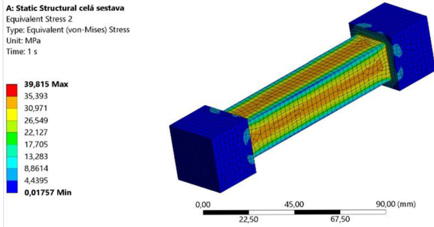
Obr. 4-8 Redukované napětí ve vzorku
