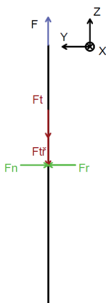
Obr. 5-5 Uvolnění hřebene
