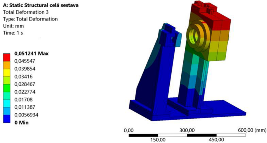
Obr. 4-6 Deformace rámu
