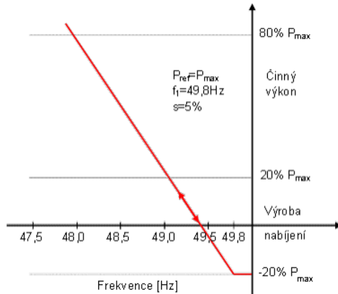
Obr zok 6.5 Ilustrat vne zn zornenie frekvennej odozvy inn ho v konu na podfrekvenciu pri akumul n ch zariadeniach [1]
