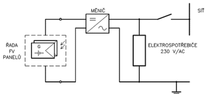
Obrázok 4.2 Bloková schéma zapojenia sieťového FVS [6]
