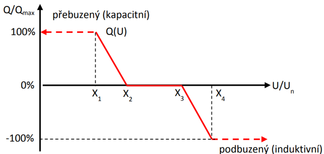
Obrázok 6.7 Charakteristická funkcia Q(U) [1]
