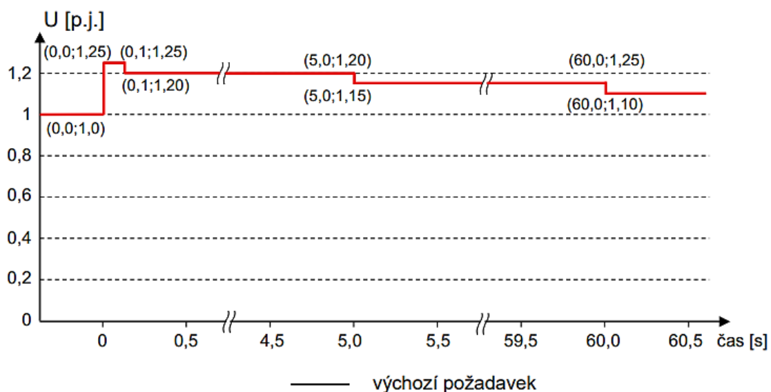
Obrázok 6.2 Schopnosť preklenutia krátkodobého nadväť pre výrobné moduly kategórie A-C [1]
