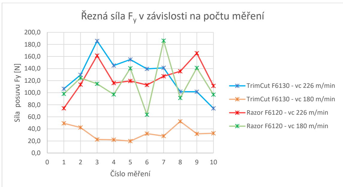
Graf 2 – Síla F_y v závislosti na počtu měřících cyklů
