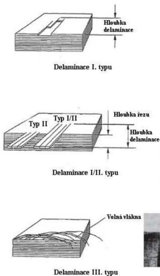
[Obr. 14] –Typy delaminací při frézování kompozitních materiálů [25]
