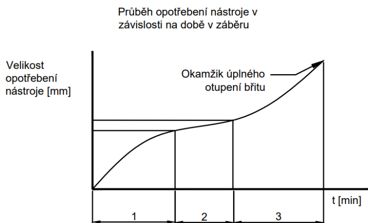
[Obr. 6] – Typický průběh opotřebení řezného nástroje
