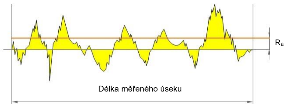
[Obr. 8] – Příklad naměřeného profilu a vyhodnocení R_a [11]
