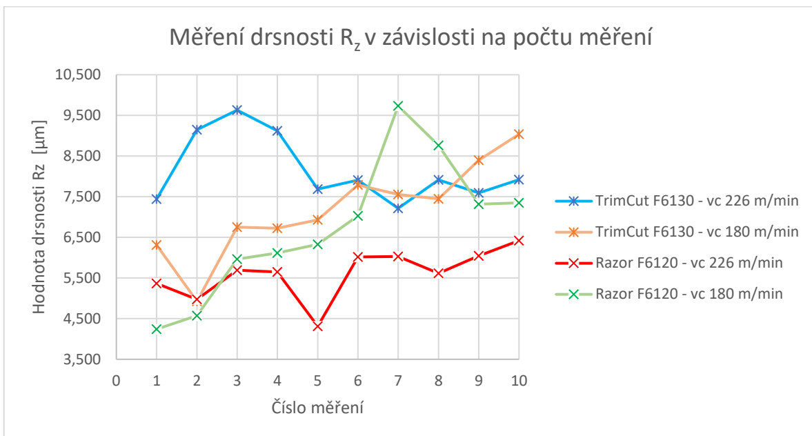
Graf 5 – Hodnota drsnosti R_z v závislosti na počtu měření
