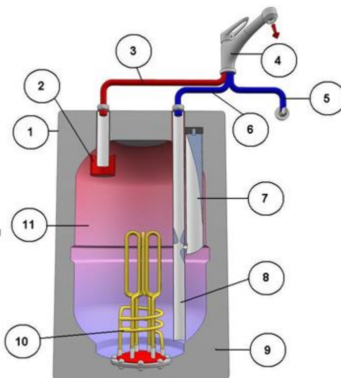
[Obr. 17 – Schéma beztlakého zásobníkového ohřivače vody, Zdroj: http://www.energetickyporadce.cz ]
