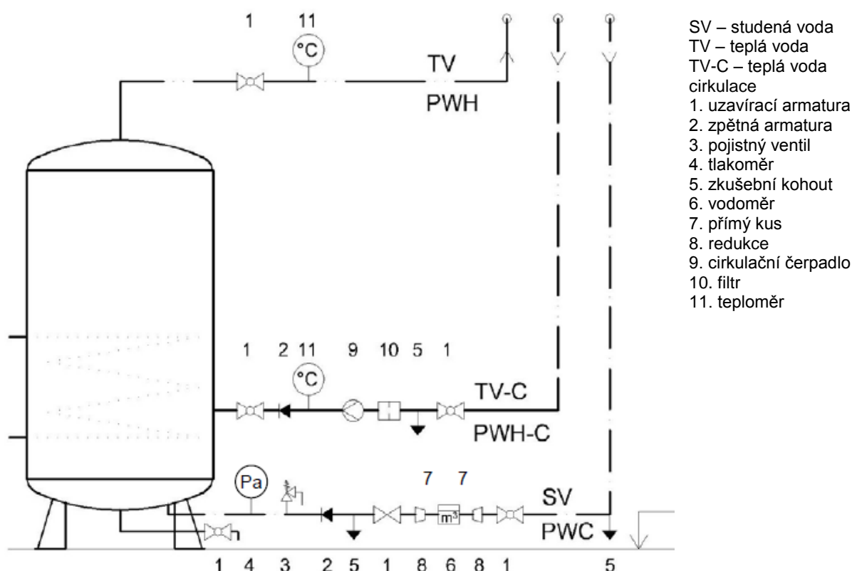
Obr. 11 – Připojení zásobníkového ohřivače – zabezpečovací zařízení, Zdroj [2]]
