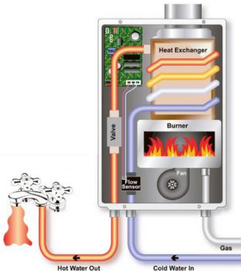
Obr. 18 – Průtokový plynový ohřivač, Zdroj: http://www.vodari.eu/voda/ohrivace-vody/prutokove-ohrivace.php
