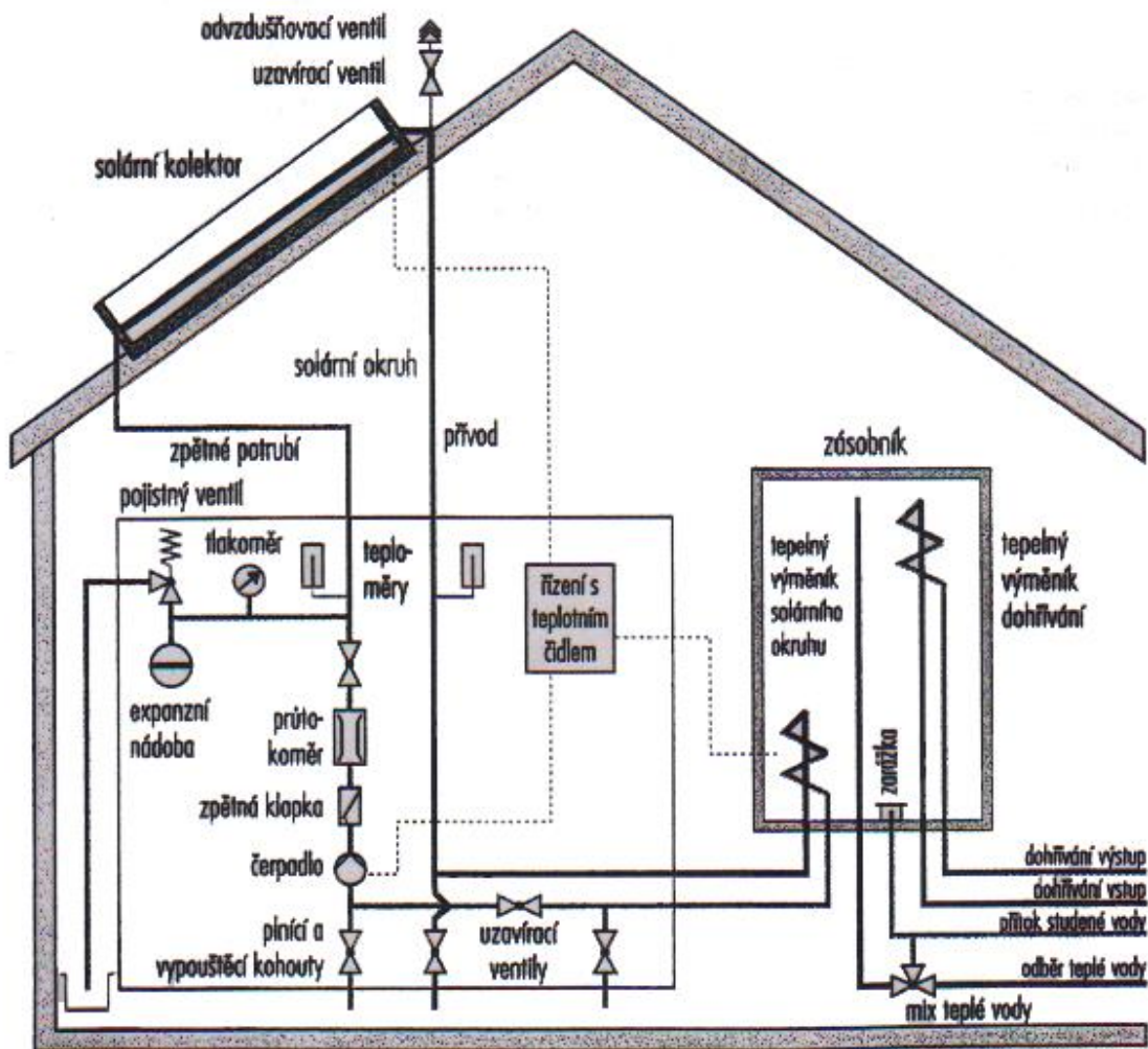
[Obr. 16 – Schéma solárního ohřevu vody, Zdroj [4]]
