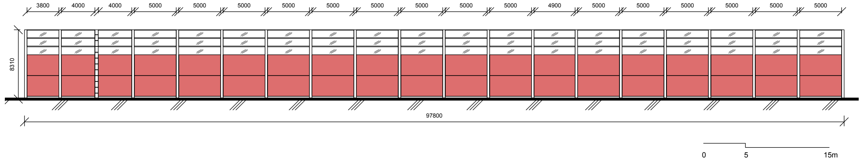
Obr. 41 Stěna B-pohled (vlastní práce)
