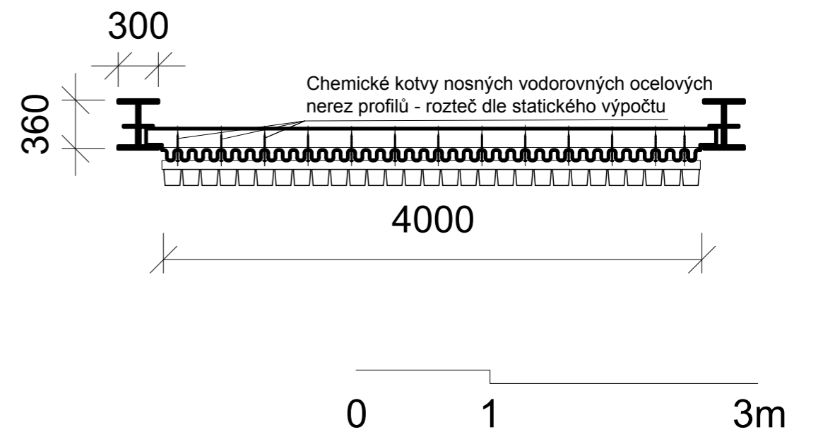
Obr. 98 Půdorys-1 pole s konstrukcí (vlastní práce)
