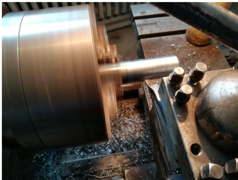
Obrázek 24 - Soustružení stopky
