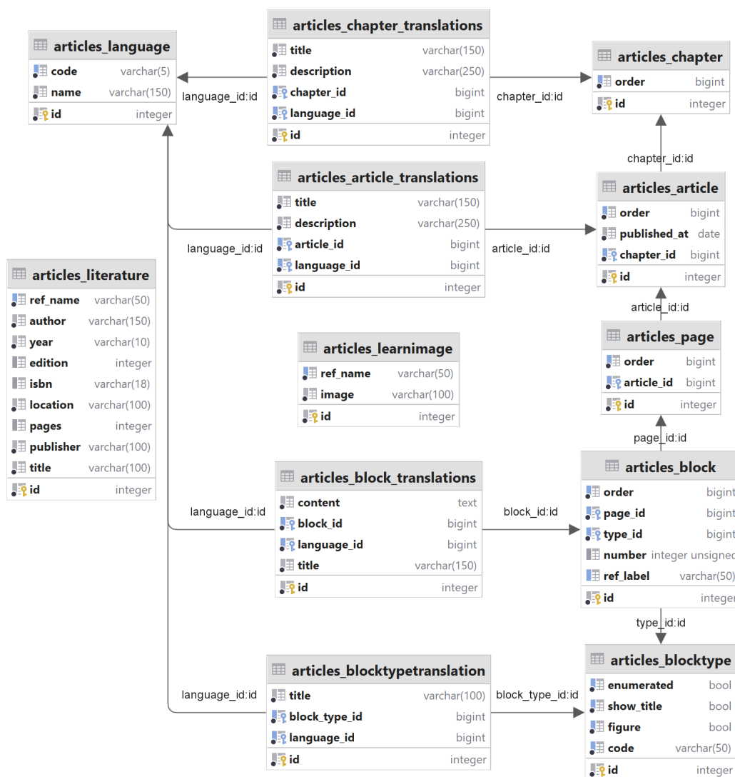
Obrázek 2: Schéma databáze
