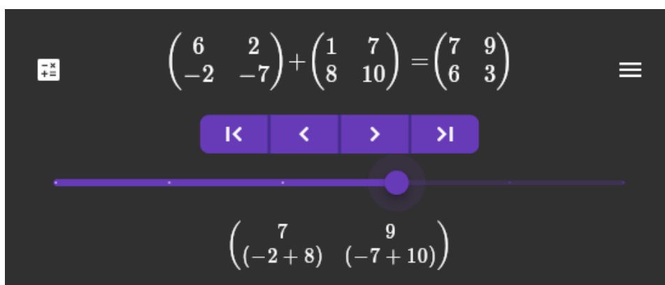
Obrázek 11: Krokování výpočtů
