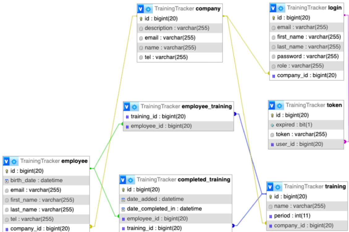
Obrázek 12: Model databáze, vlastní zpracování v phpMyAdmin
