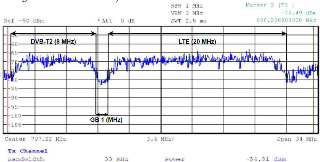
Obr. 3 Zobrazení obou spekter na FSQ analyzátoru pro B_{LTE} 20 MHz
