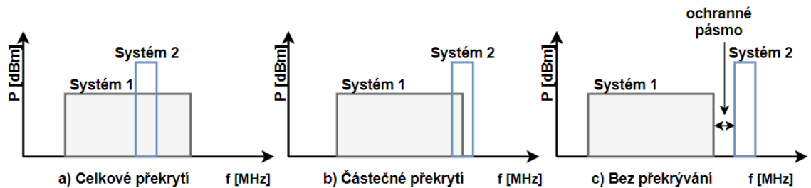
Obr. 3.3 Typy koexistenčních scénářů
