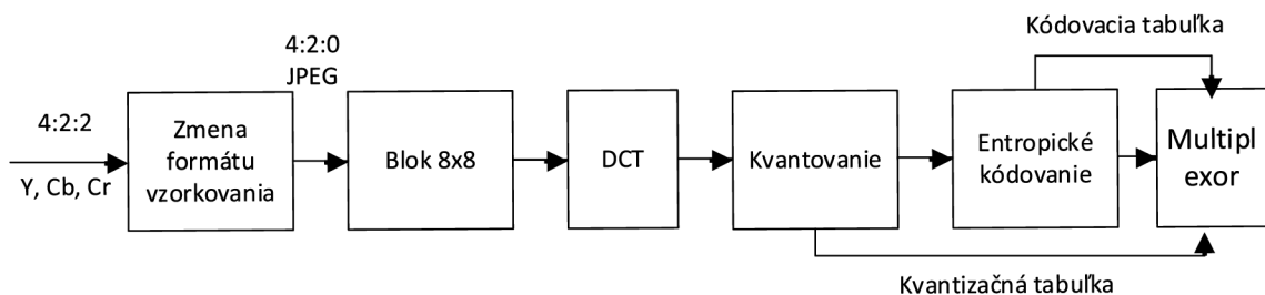
Obr. 2.1: Schéma kódovania JPEG
