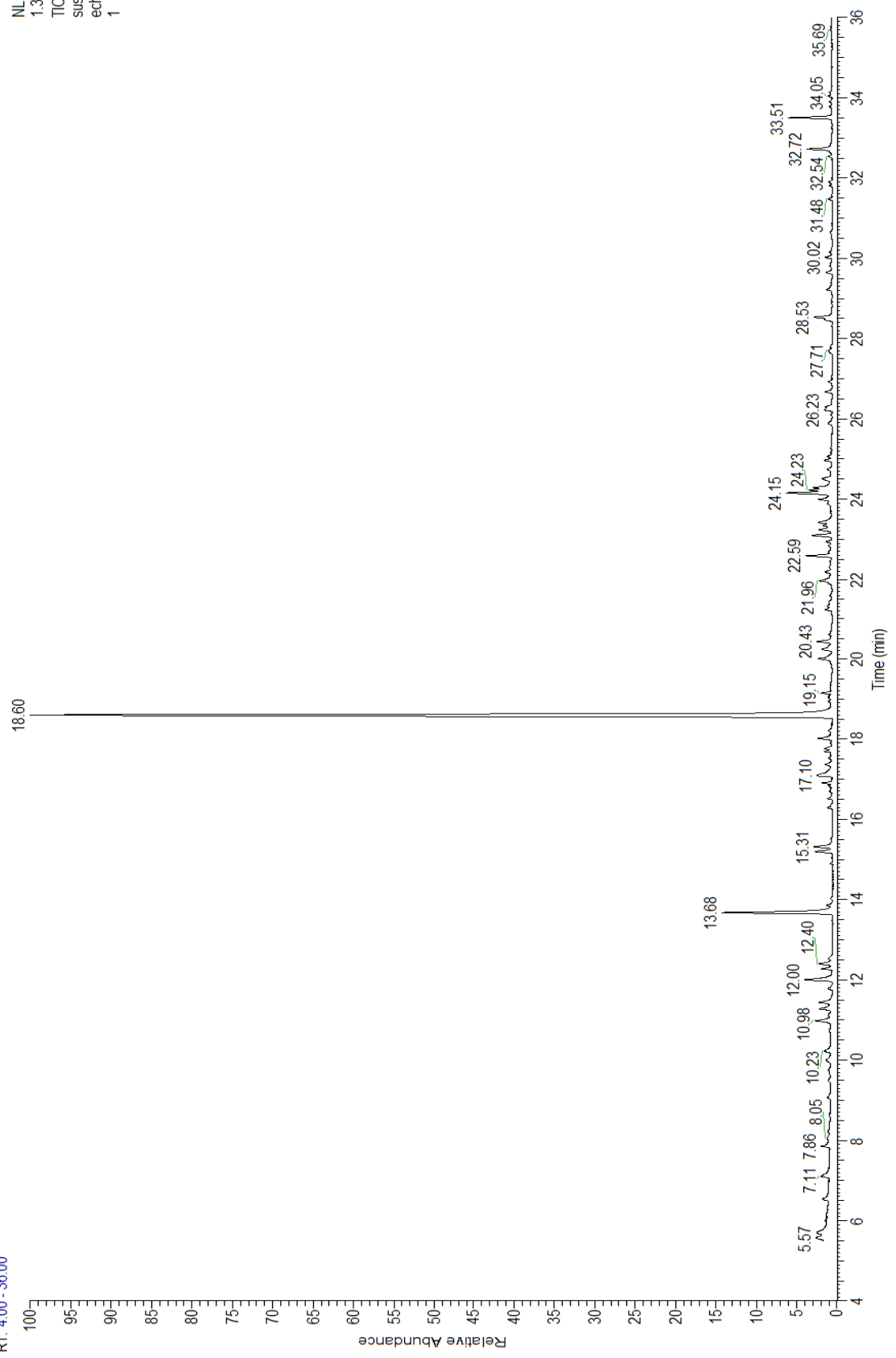
Příloha 4 Chromatogram sušené echinacey ( Echinacea purpurea )
