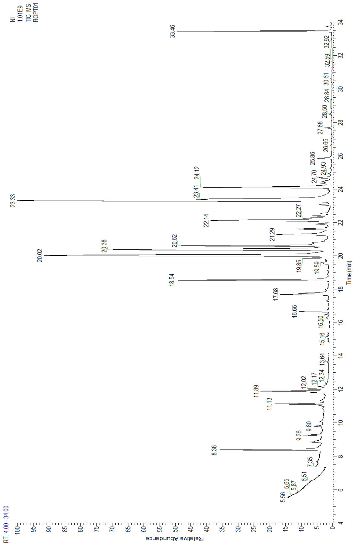
Příloha 5 Chromatogram extraktu rýmovníku ( Plectranthus amboinicus )
