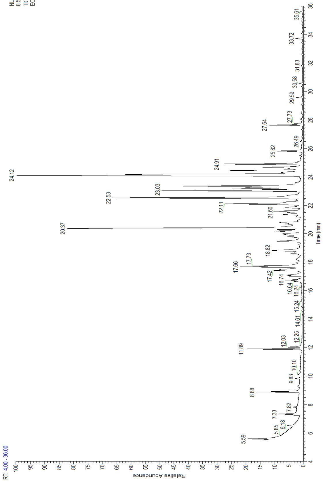
Příloha 6 Chromatogram extraktu echinacey ( Echinacea purpurea )
