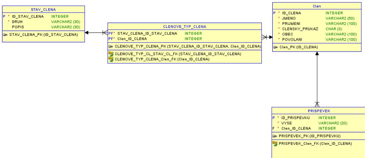
Příloha č. 15, Relační model přiložené databáze členů Družstva pro vystavení Kodymova národního domu
