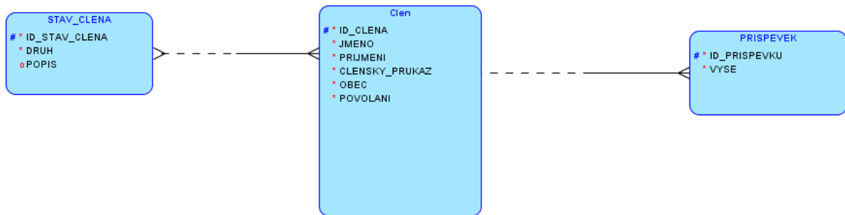
Příloha č. 14, Logický model přiložené databáze členů Družstva pro vystavení Kodymova národního domu
