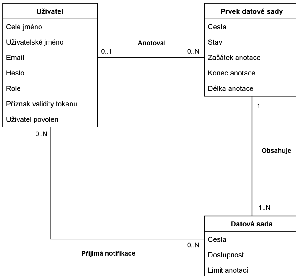
Obrázek 3.6: Schéma databáze.
