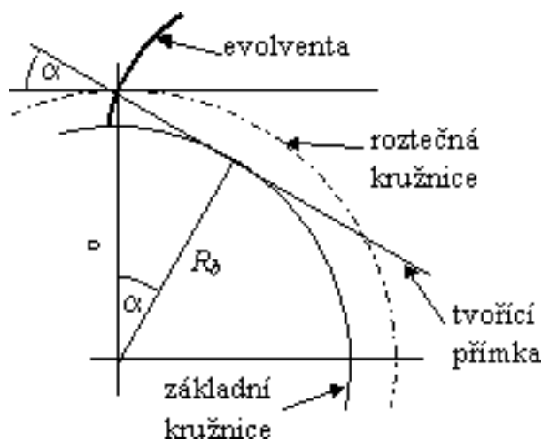
Obr. 2.3 Evolventa [10].
