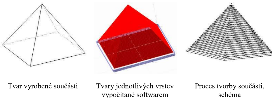
Obr. 3.1 Obecný princip technologie RP [14].
