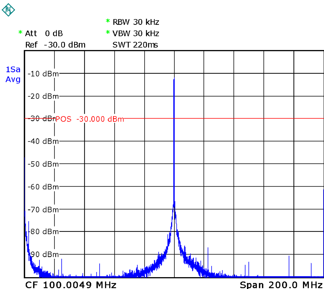
Obr. 1.12: Širokopásmové spektrum generovaného stálého kmitočtu.
