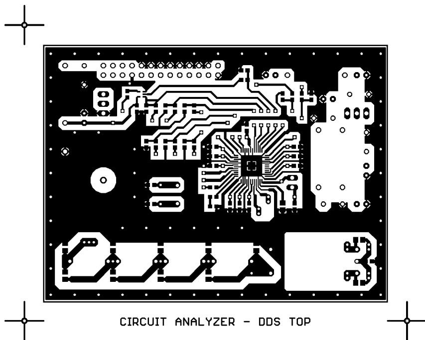
Obrazec horní vrstvy (měřítko 1:1).
