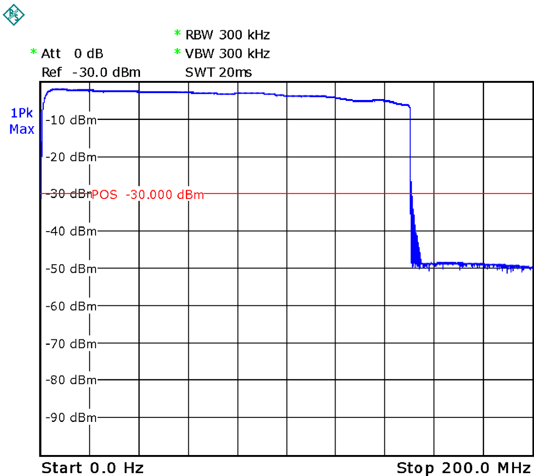
Obr. 1.13: Závislost výstupní úrovně na kmitočtu generovaného signálu.
