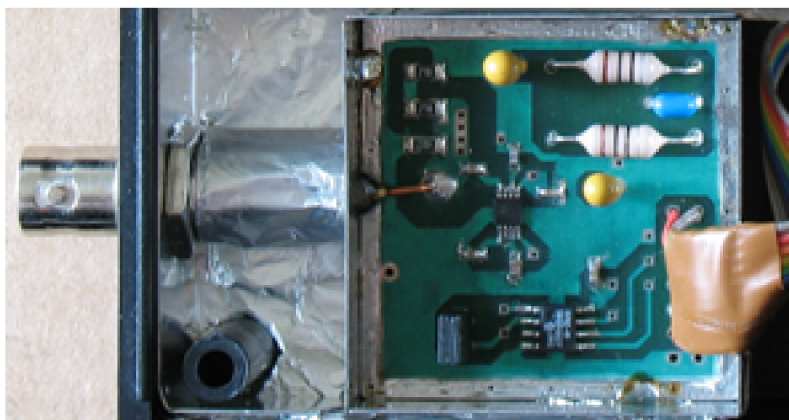
Obr. 1.14: Fotografie logaritmického detektoru.
