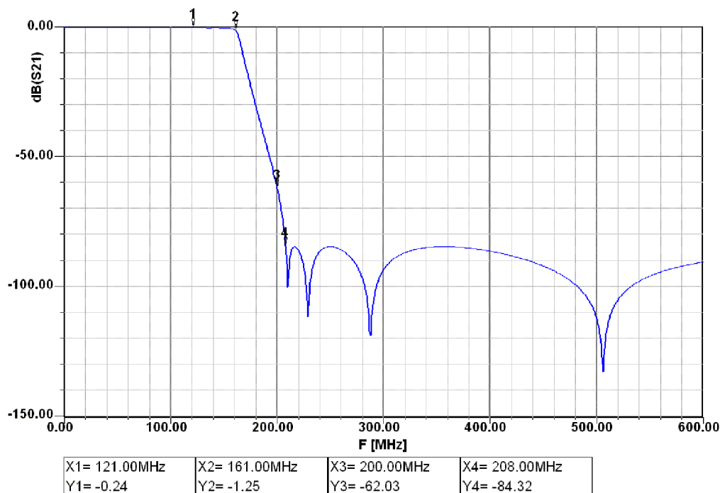
Obr. 1.4: Přenos idealizovaného rekonstrukčního filtru.
