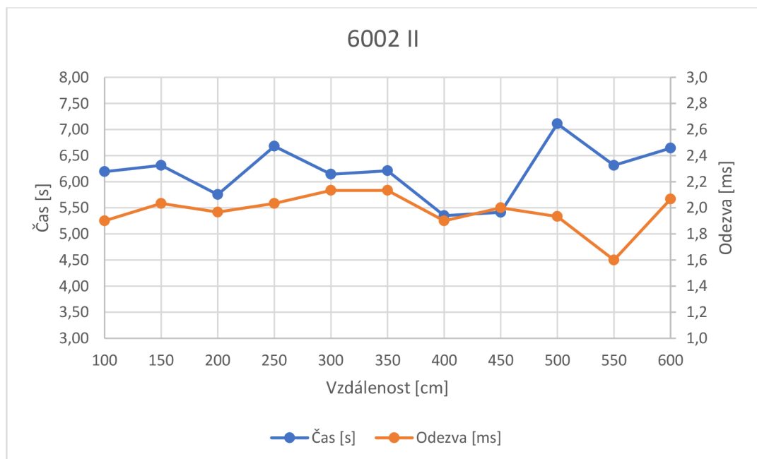
Graf 2 odezva a čas při opětovném připojení Trulifi 6002 (Zdroj: (vlastní))
