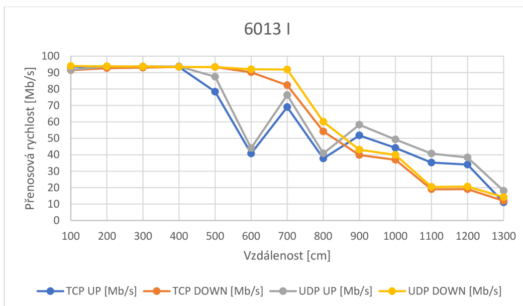
Graf 3 Přenosové rychlosti v závislosti na vzdálenosti Trulifi 6013 (Zdroj: (vlastní))
