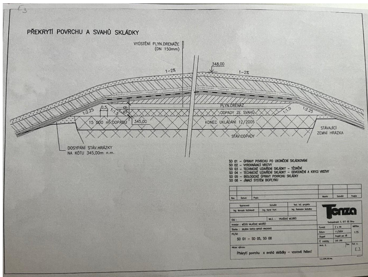
Obr. 17 Překrytí povrchu a svahů skládky – Tenza (obec Krhová)
